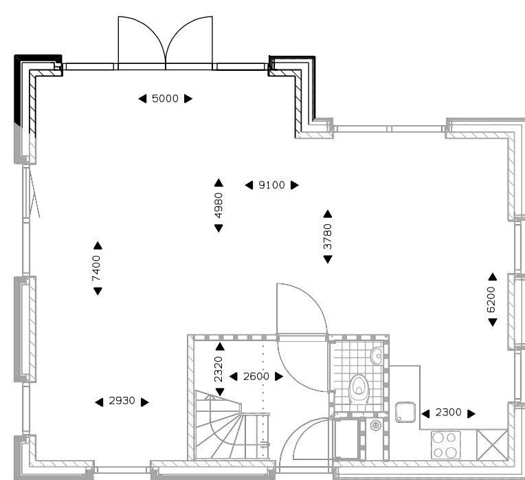
Begane grond uitbouw 1200mm. dubbele tuindeur.
