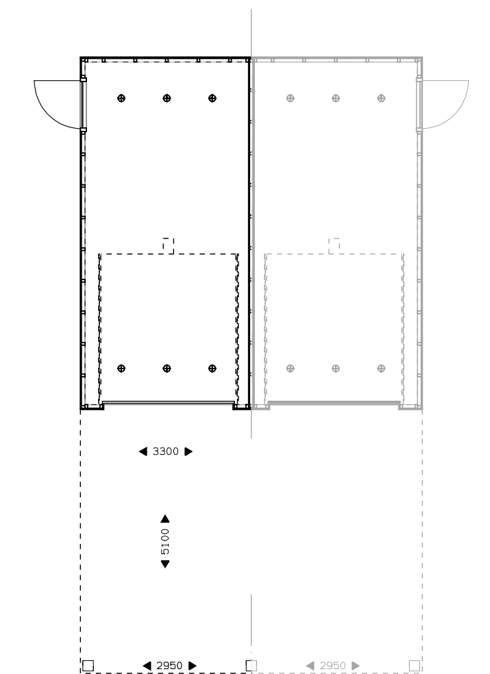
Begane grond uitbouw 2400mm. elektrisch bedienbare sectionaaldeur. natuurlijke ventilatie.
