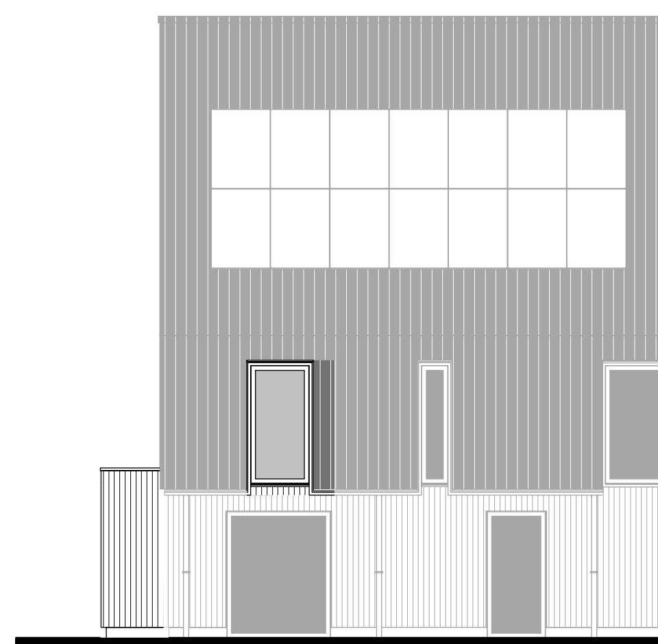
Zijgevel links uitbouw 1200mm. bij vergroten badkamer.
