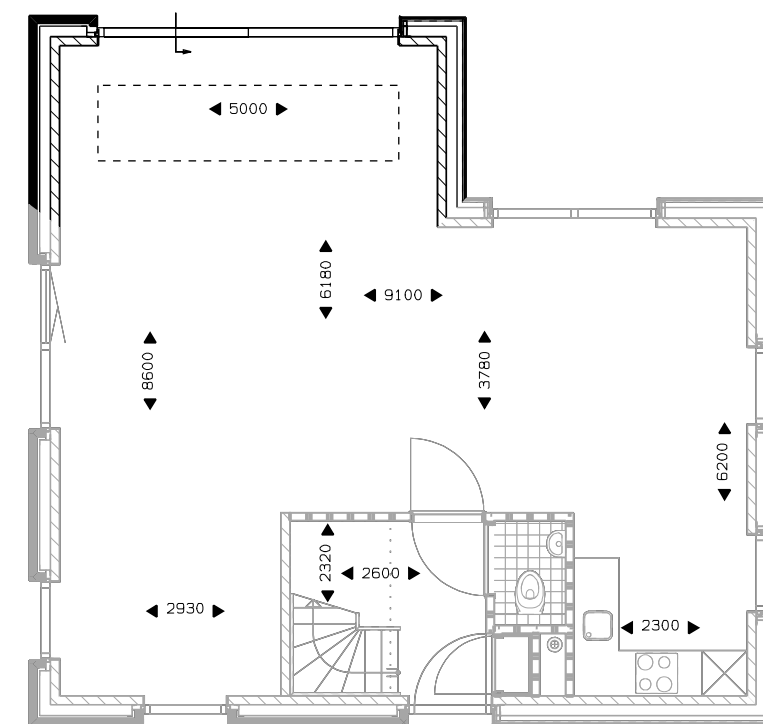
Begane grond uitbouw 2400mm. schuifpui. lichtstraat 3 vlakken 2,40x1 m. lichtstraat 4 vlakken 3,19x1 m. lichtstraat 5 vlakken 3,89x1 m.
