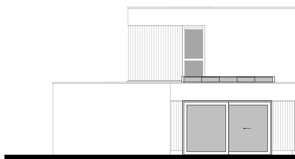
Achtergevel schuifpui. lichtstraat 3 vlakken 2,40x1 m. lichtstraat 4 vlakken 3,19x1 m. lichtstraat 5 vlakken 3,89x1 m.
