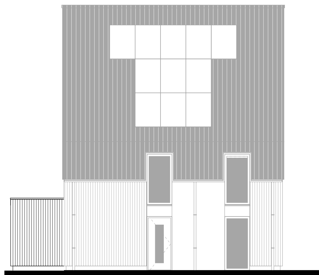
Zijgevel links uitbouw 2400mm.
