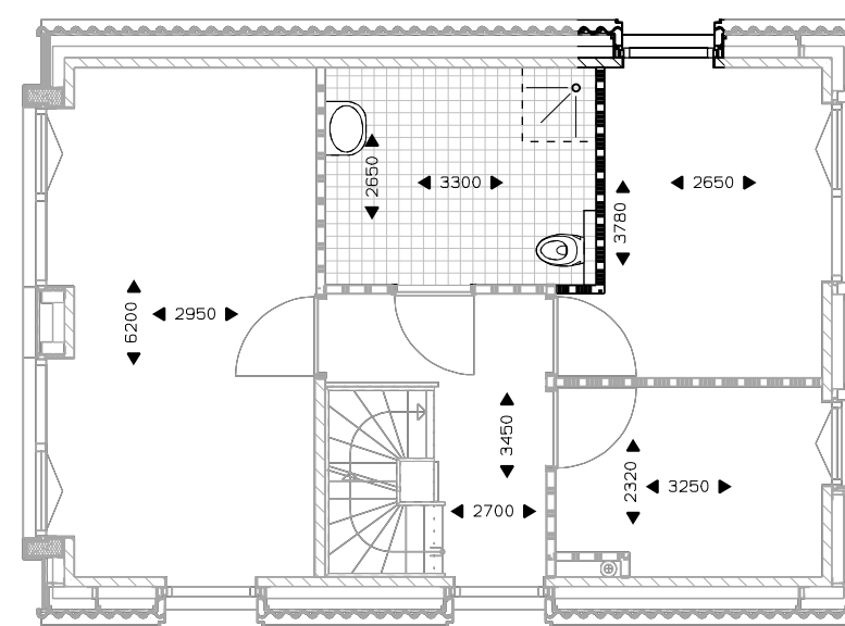
Verdieping 1 vergroten badkamer met 60 cm.
