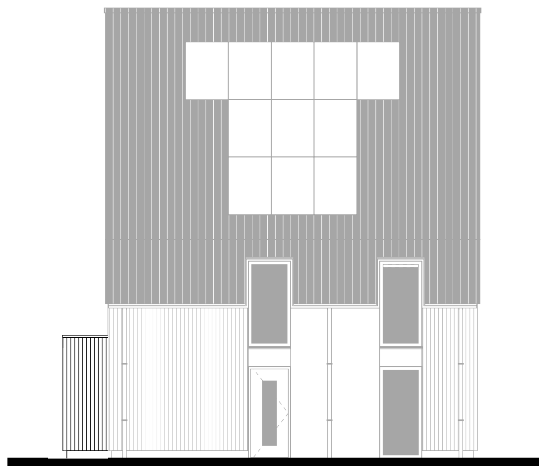
Zijgevel links uitbouw 1200mm.
