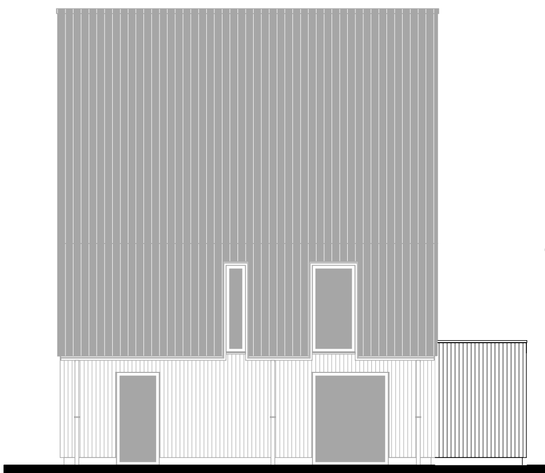
Zijgevel rechts uitbouw 2400mm.
