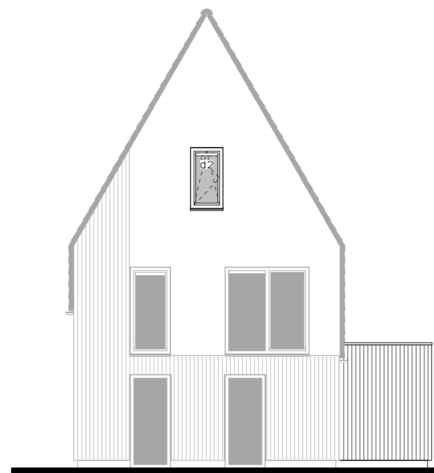
Achtergevel uitbouw 2400mm.
