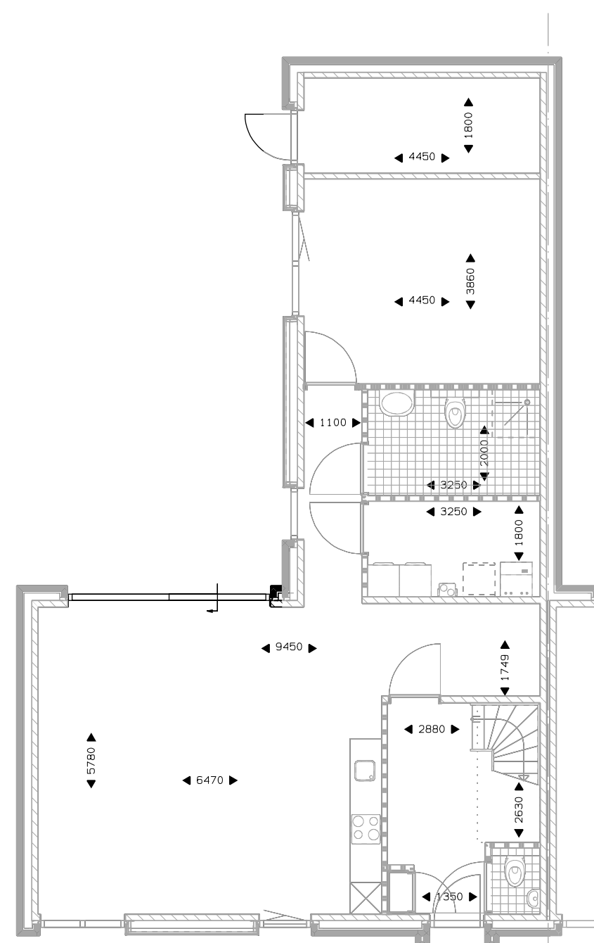
Begane grond schuifpui.
