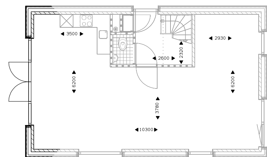
Begane grond uitbouw 1200mm. dubbele tuindeur.
