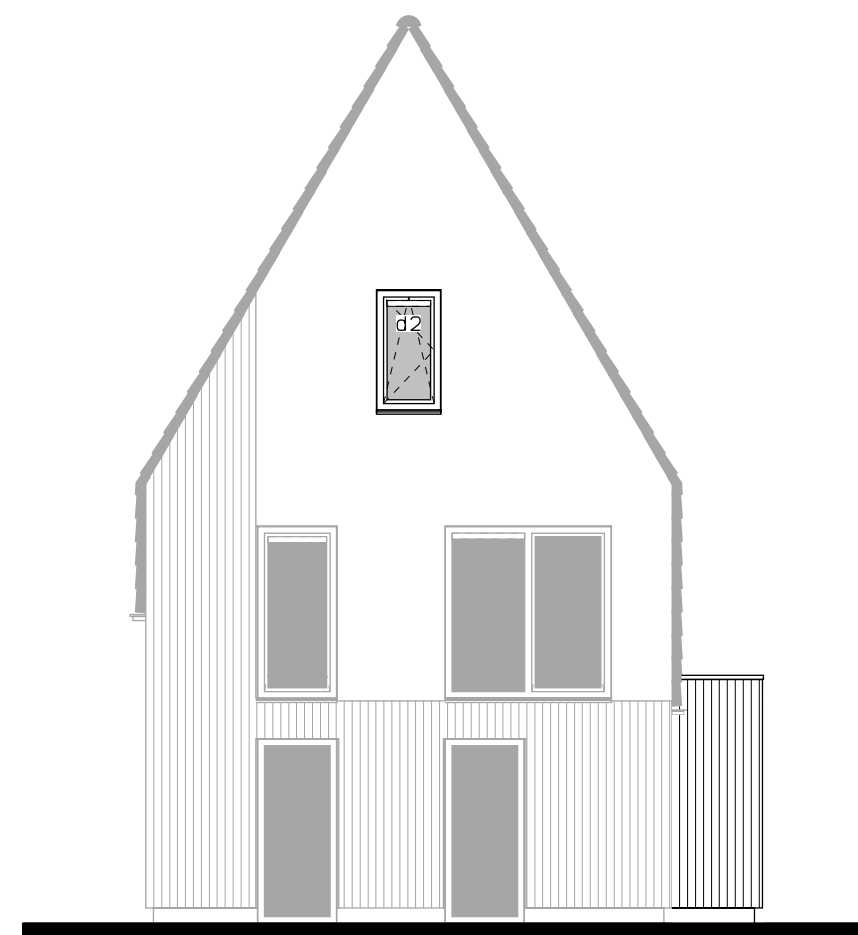
Achtergevel uitbouw 1200mm.
