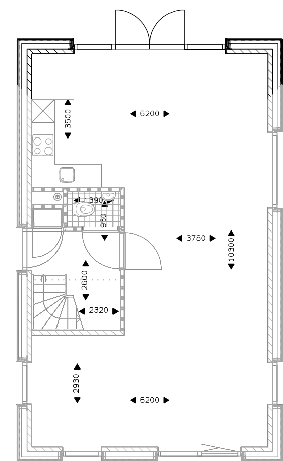
Begane grond uitbouw 1200mm. dubbele tuindeur.
