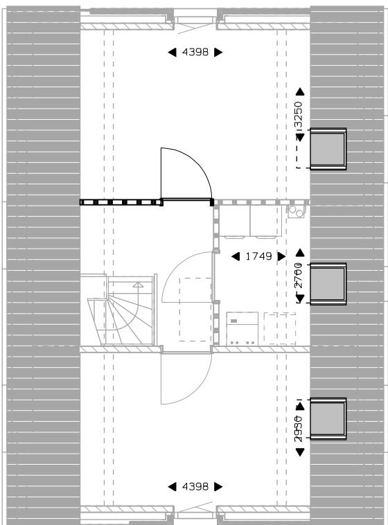
Verdieping 2 slaapkamer. dakvenster. sparing dakvenster.
