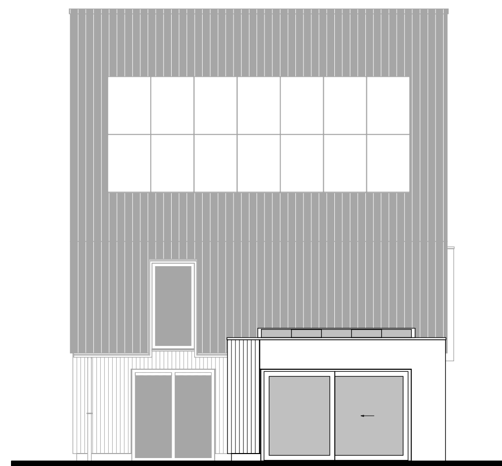
Zijgevel links uitbouw 2400mm. schuifpui. lichtstraat 3 vlakken 2,40x1 m. lichtstraat 4 vlakken 3,19x1 m. lichtstraat 5 vlakken 3,89x1 m.
