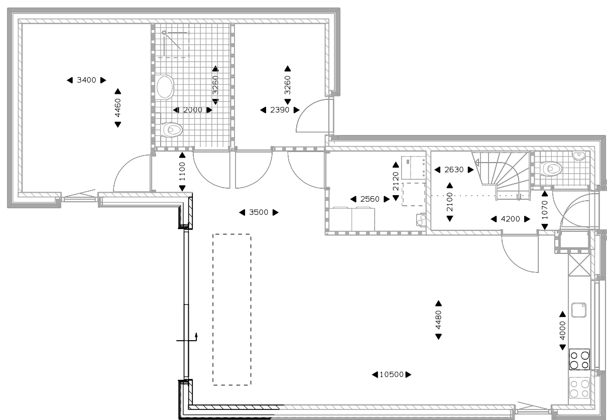
Begane grond uitbouw 2400mm. schuifpui. lichtstraat 3 vlakken 2,40x1 m. lichtstraat 4 vlakken 3,19x1 m. lichtstraat 5 vlakken 3,89x1 m.
