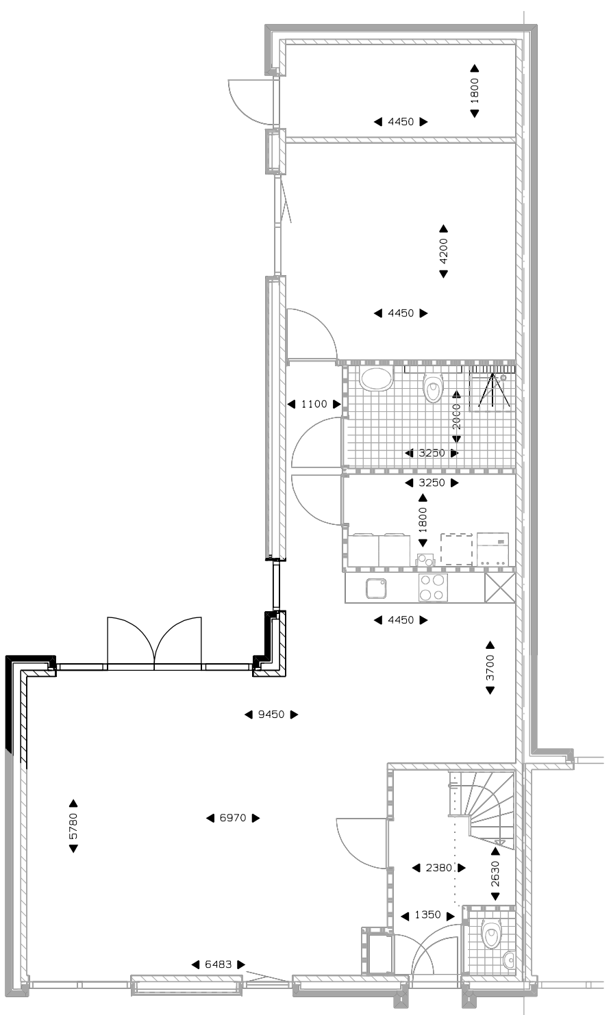
Begane grond uitbouw 1800mm. dubbele tuindeur.
