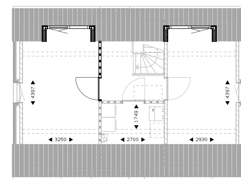
Verdieping 2 slaapkamer. dakkapel (max. 1/dakvlak). sparing dakkapel (max. 1/dakvlak).
