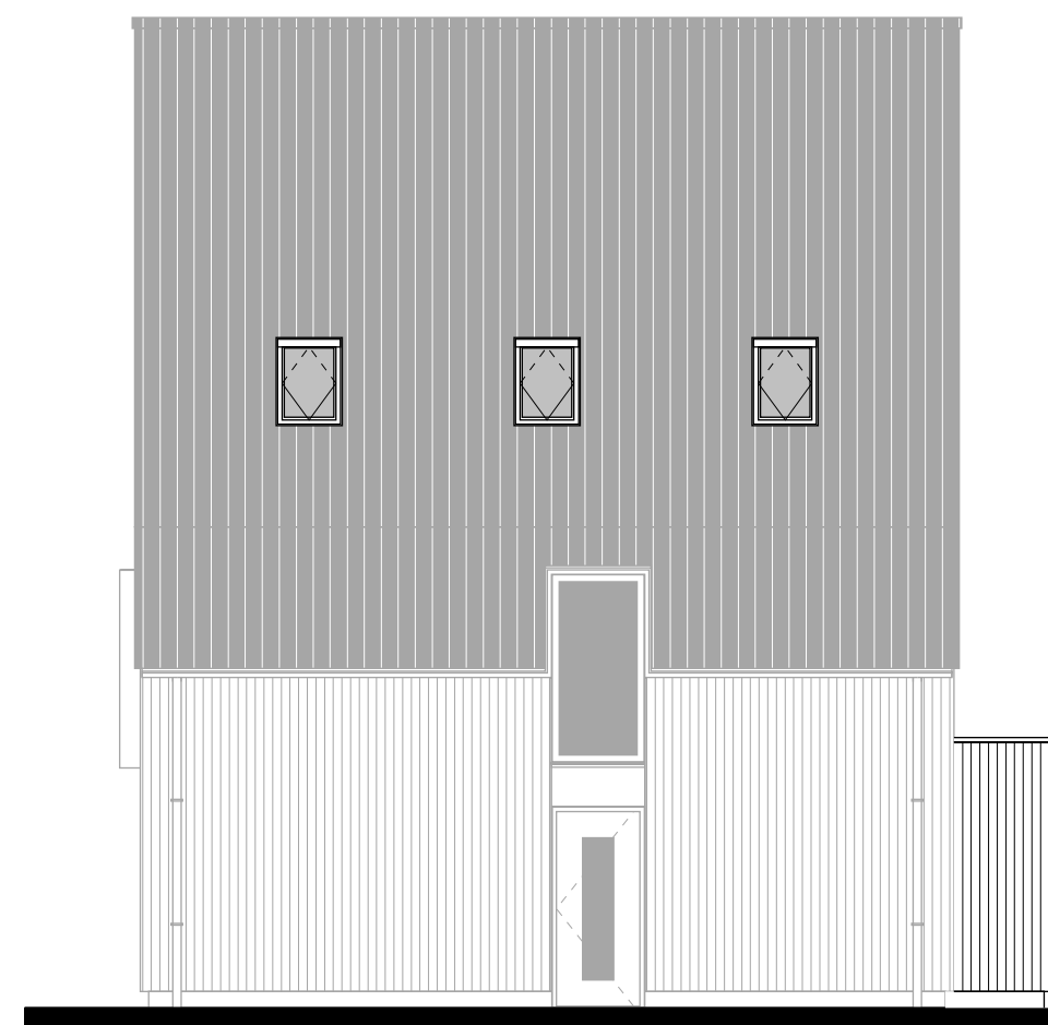
Zijgevel rechts uitbouw 1200mm. dakvenster. sparing dakvenster.
