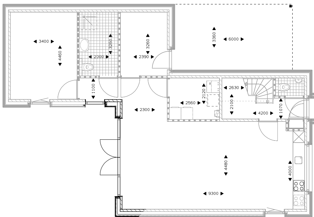
Begane grond uitbouw 1200mm. dubbele tuindeur. carport.
