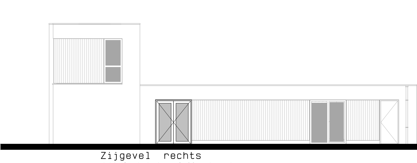
Zijgevel rechts dubbele tuindeur 2,00 m breed.
