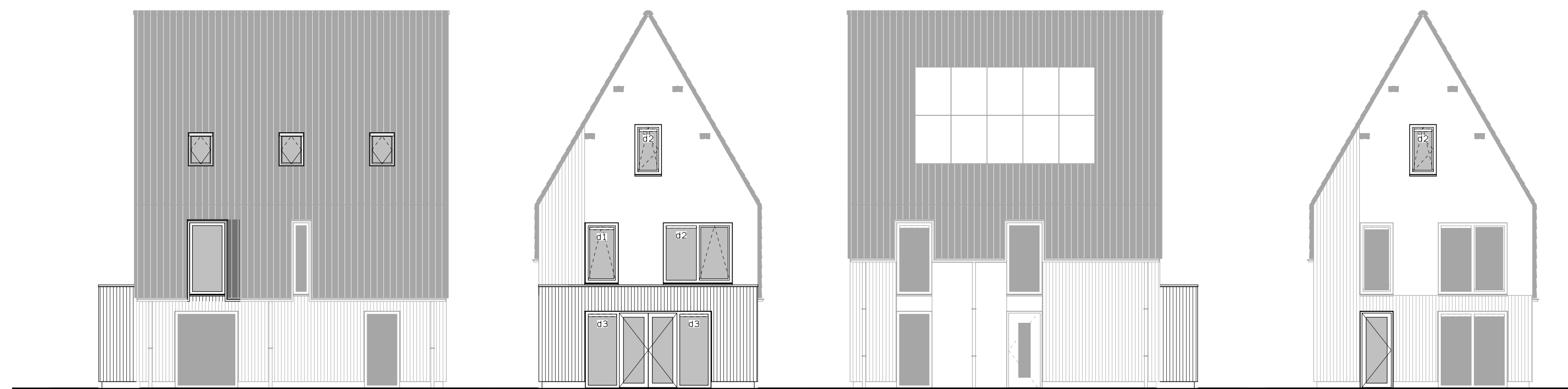
Zijgevel links uitbouw 1200mm. bij vergroten badkamer. dakvenster. sparing dakvenster.
