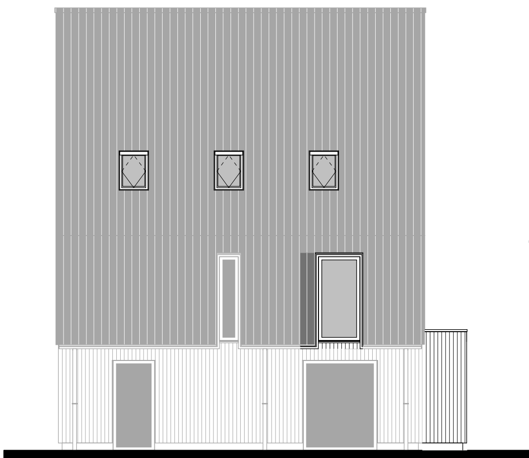
Zijgevel rechts uitbouw 1200mm. bij vergroten badkamer. dakvenster. sparing dakvenster.
