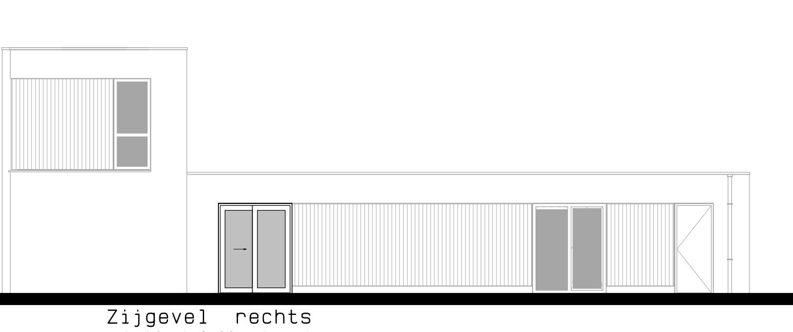
Zijgevel rechts schuifpui 2,00 m breed.
