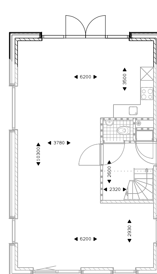
Begane grond uitbouw 1200mm. dubbele tuindeur.
