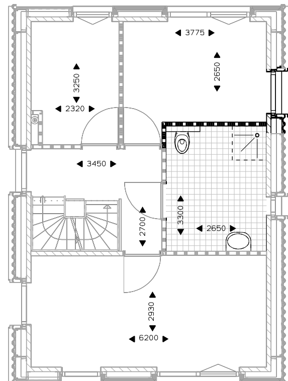
Verdieping 1 vergroten badkamer met 60 cm.
