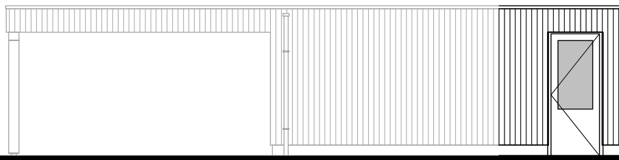
Zijgevel rechts uitbouw 2400mm. glasopening borstwering ca. 90 cm.
