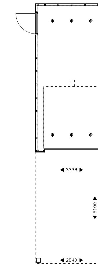
Begane grond uitbouw 2400mm. elektrisch bedienbare sectionaaldeur. natuurlijke ventilatie.
