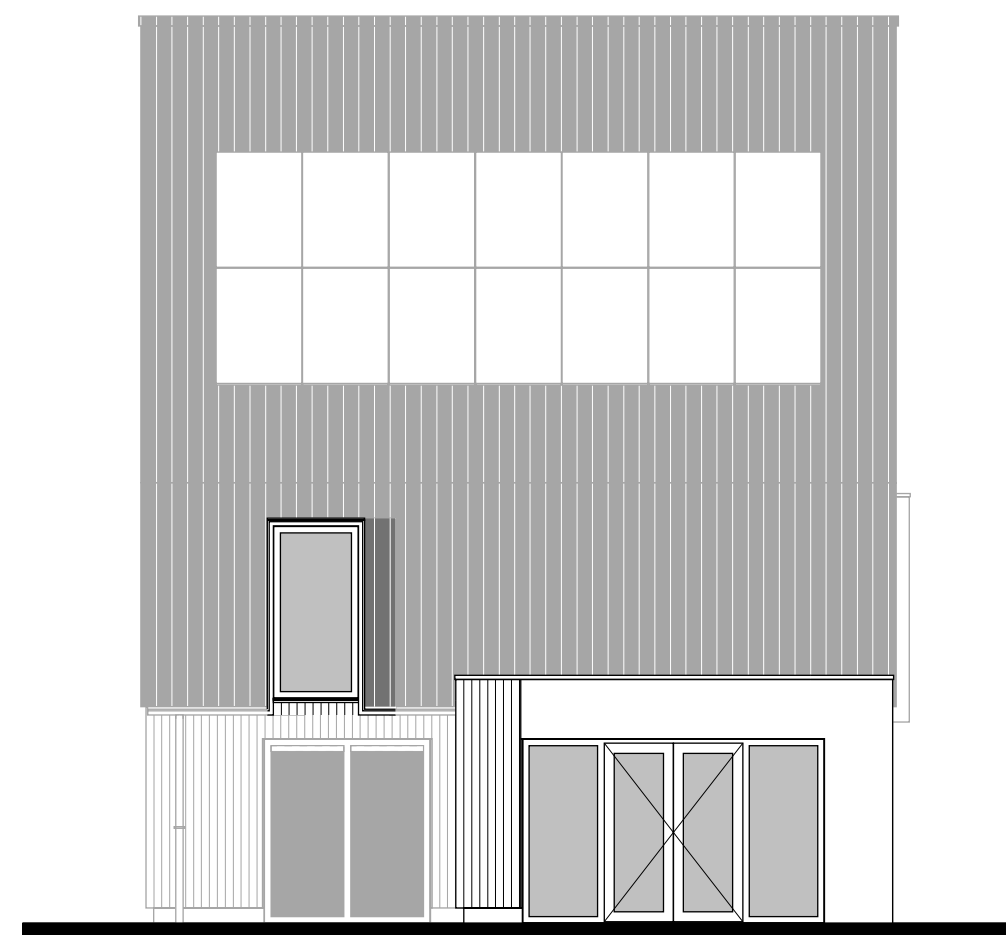
Zijgevel links uitbouw 1200mm. dubbele tuindeur. bij vergroten badkamer.
