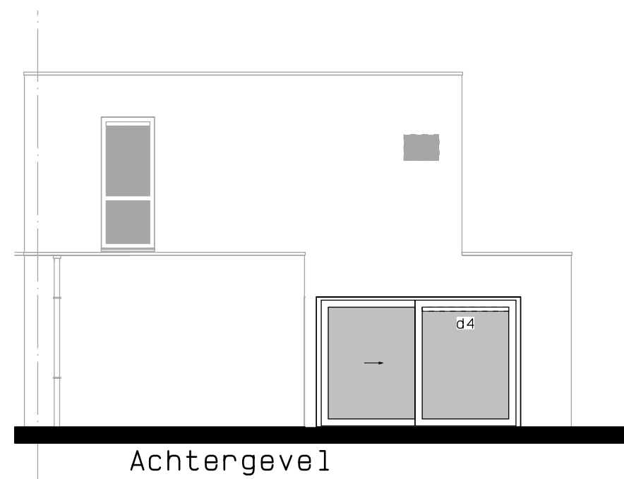
Achtergevel schuifpui.
