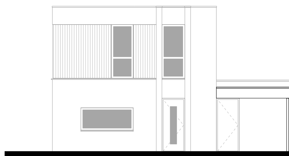
Voorgevel carport
