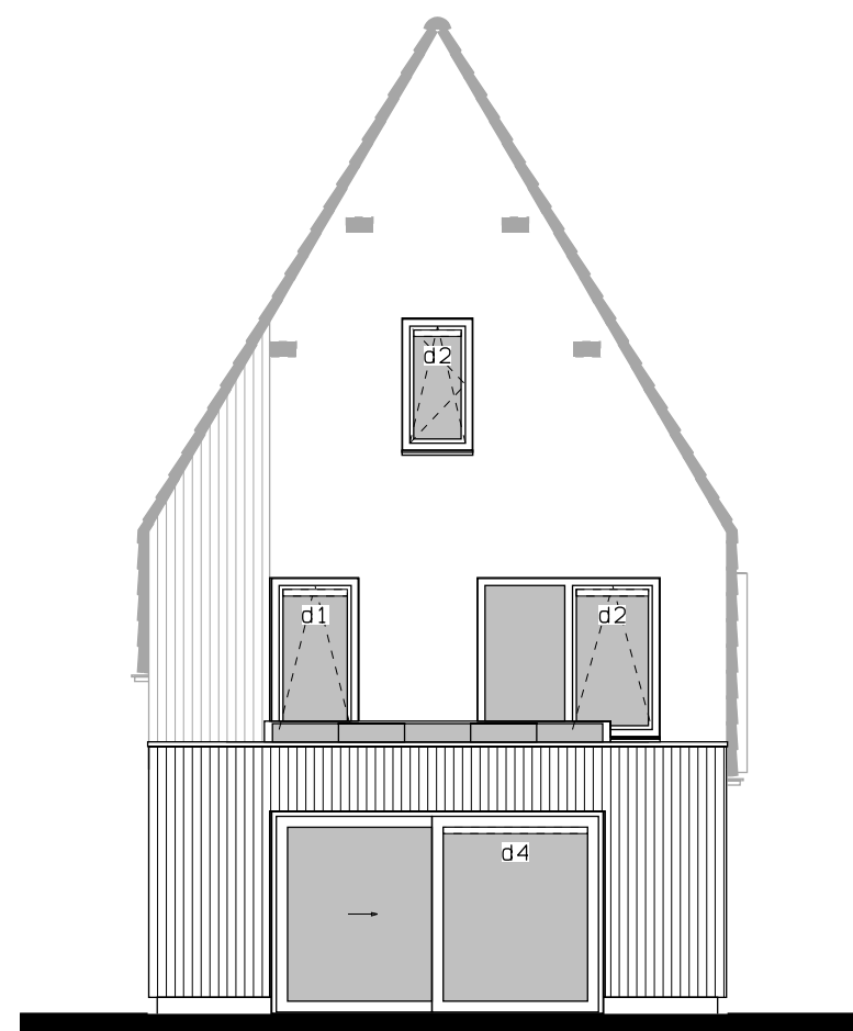
Achtergevel uitbouw 2400mm. schuifpui. lichtstraat 3 vlakken 2,40x1 m. lichtstraat 4 vlakken 3,19x1 m. lichtstraat 5 vlakken 3,89x1 m.
