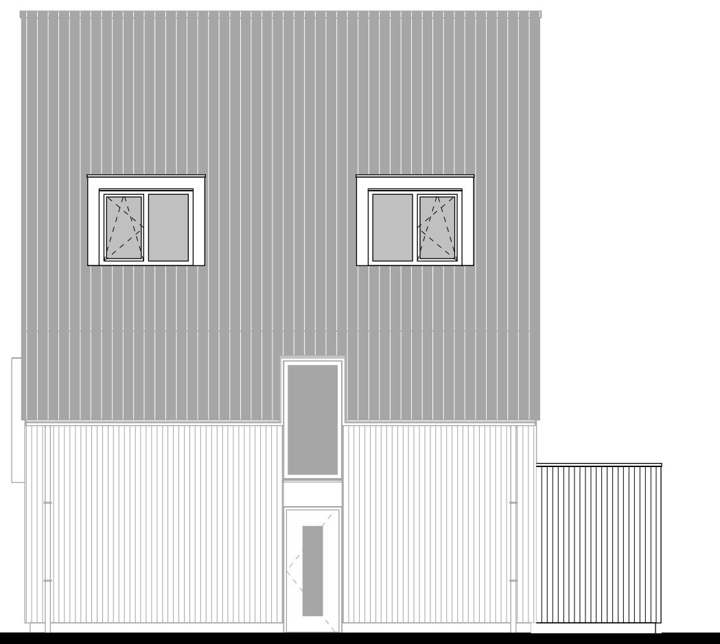
Zijgevel rechts uitbouw 2400mm. dakkapel (max. 1/dakvlak). sparing dakkapel (max. 1/dakvlak).
