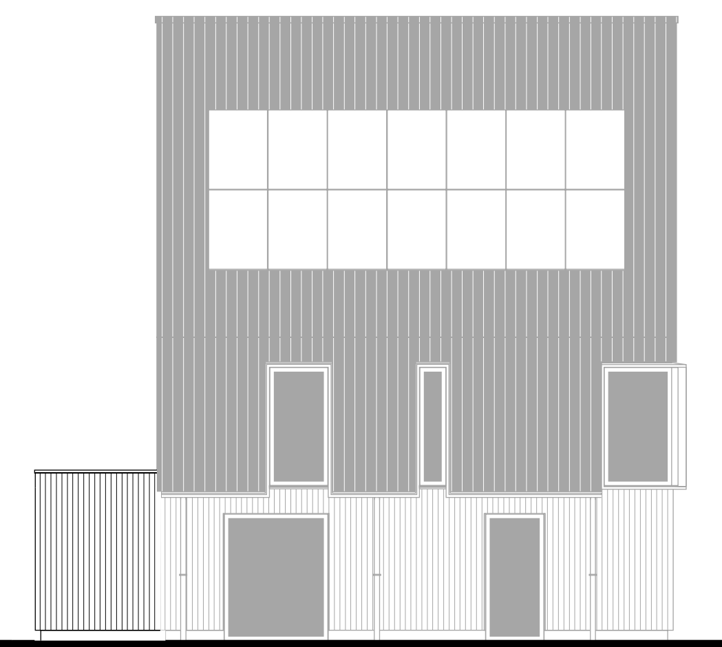
Zijgevel links uitbouw 2400mm.
