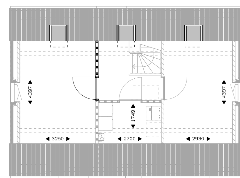
Verdieping 2 slaapkamer. dakvenster. sparing dakvenster.
