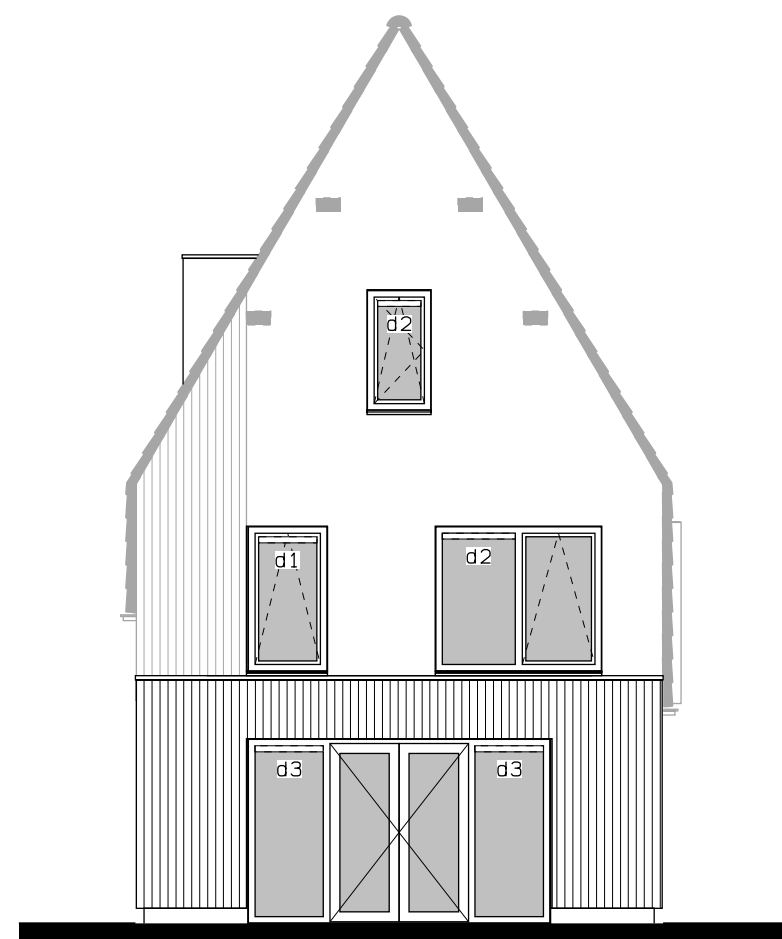
Achtergevel uitbouw 1200mm. dubbele tuindeur. dakkapel.
