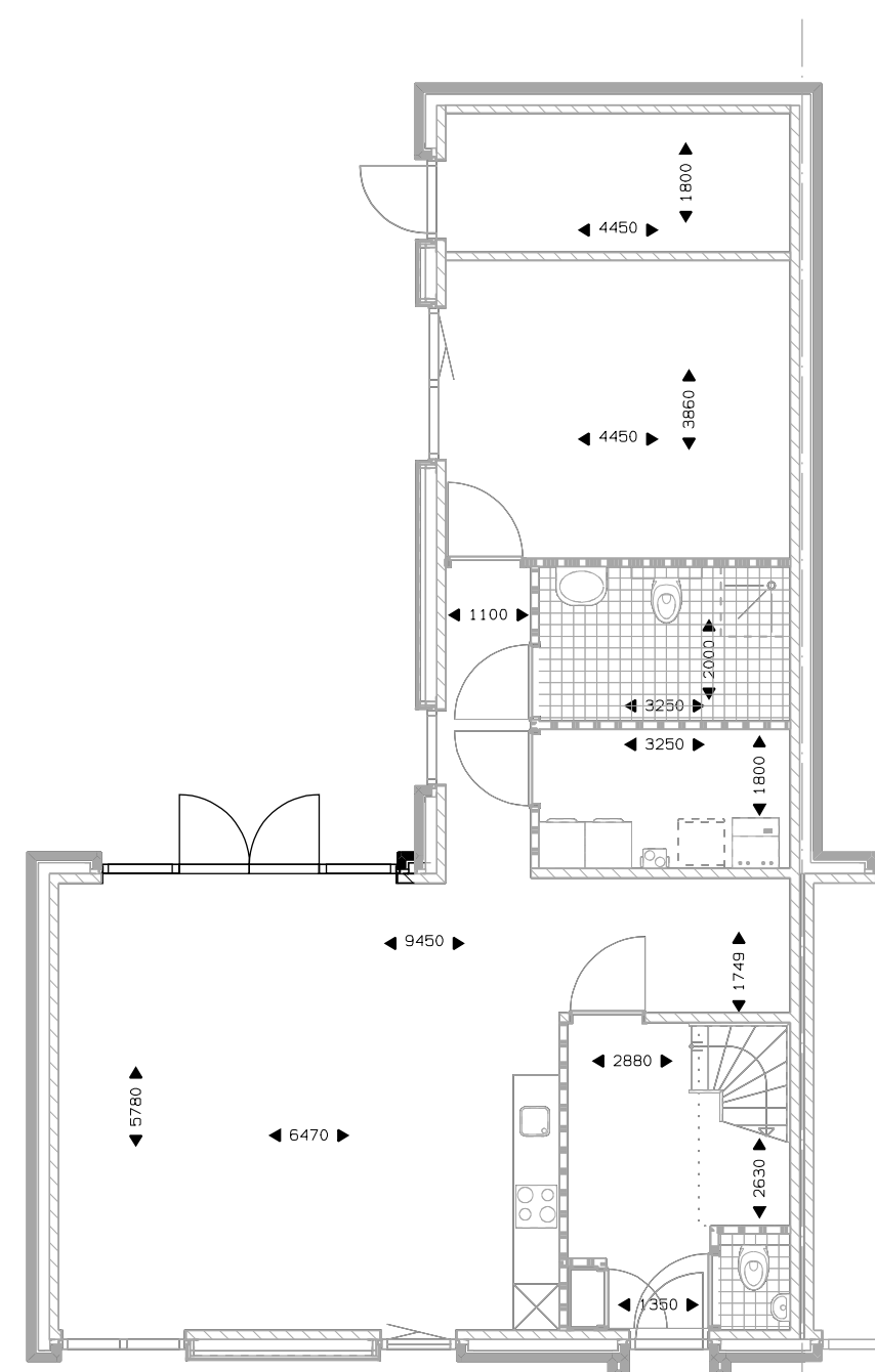
Begane grond dubbele tuindeur.
