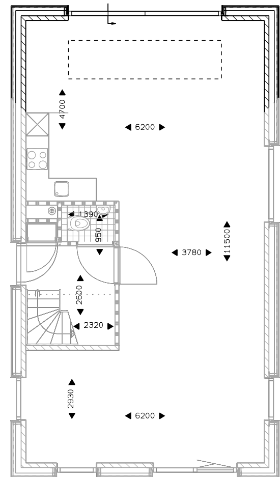
Begane grond uitbouw 2400mm. schuifpui. lichtstraat 3 vlakken 2,40x1 m. lichtstraat 4 vlakken 3,19x1 m. lichtstraat 5 vlakken 3,89x1 m.
