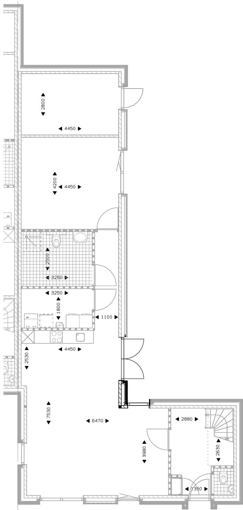
Begane grond dubbele tuindeur 2,00 m breed.
