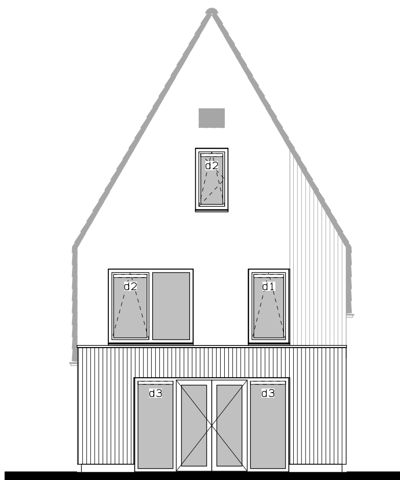
Achtergevel uitbouw 1200mm. dubbele tuindeur.
