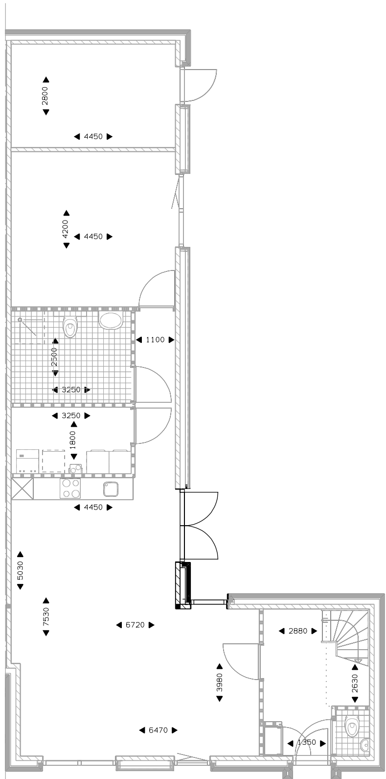
Begane grond dubbele tuindeur 2,00 m breed.
