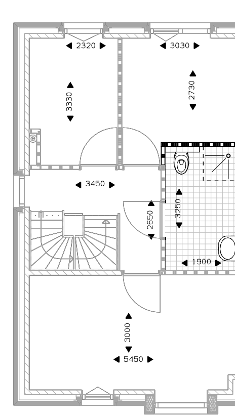
verdieping 1 vergroten badkamer met 60 cm.
