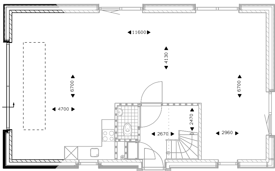
Begane grond uitbouw 2400mm *. schuifpui. lichtstraat 3 vlakken 2,40x1 m. lichtstraat 4 vlakken 3,19x1 m. lichtstraat 5 vlakken 3,89x1 m.
