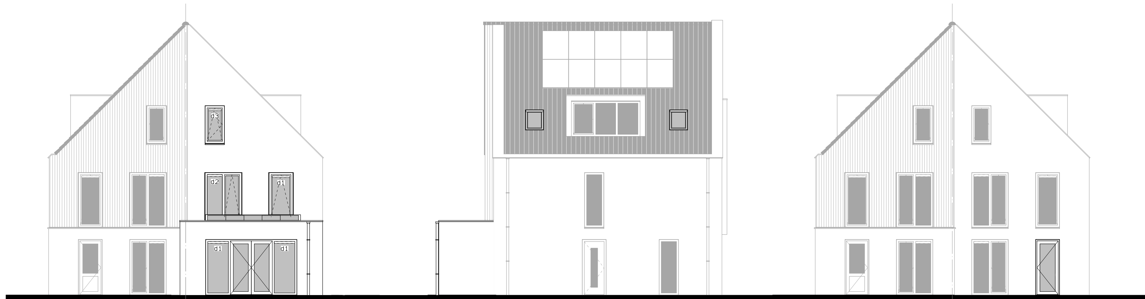
Achtergevel uitbouw 2400mm. dubbele tuindeur. lichtstraat 3 vlakken 2,40x1 m. lichtstraat 4 vlakken 3,19x1 m. lichtstraat 5 vlakken 3,89x1 m.
