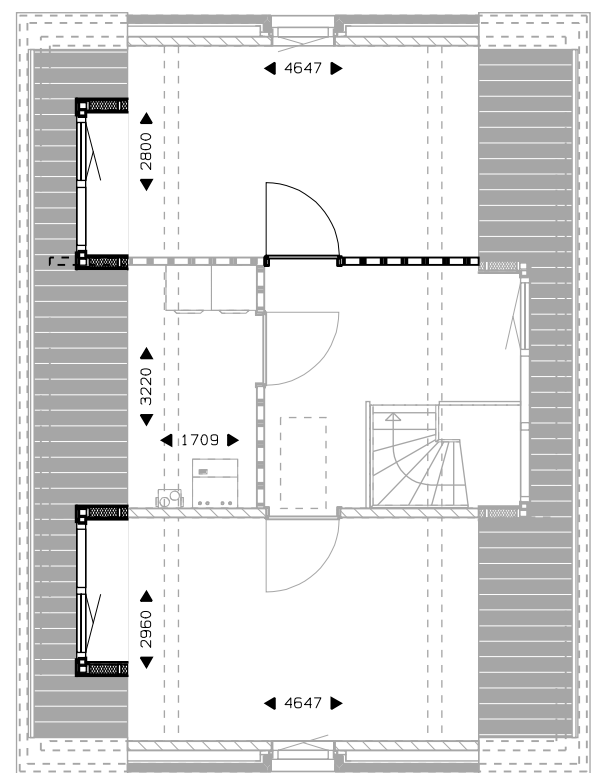
Verdieping 2 slaapkamer. dakkapel (max. 1/dakvlak). sparing dakkapel (max. 1/dakvlak).
