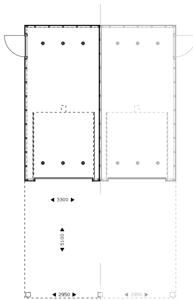
Begane grond uitbouw 2400mm. elektrisch bedienbare sectionaaldeur. natuurlijke ventilatie.
