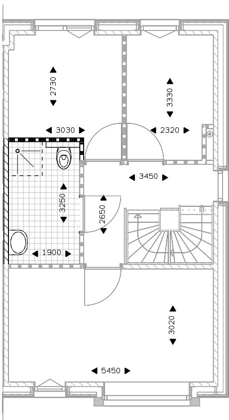
verdieping 1 vergroten badkamer met 60 cm.
