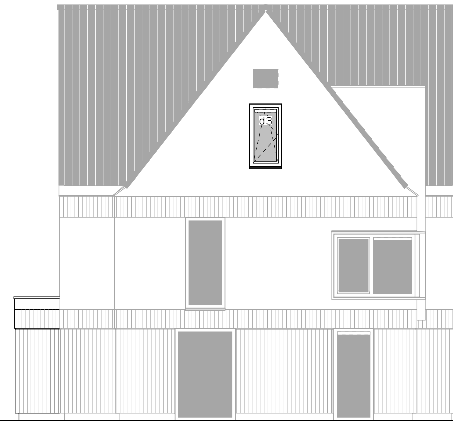
Zijgevel links uitbouw 1200mm.
