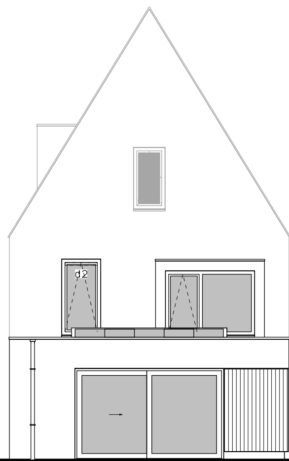
Achtergevel uitbouw 2400mm *. schuifpui. deur lage borstwering. lichtstraat 3 vlakken 2,40x1 m. lichtstraat 4 vlakken 3,19x1 m. lichtstraat 5 vlakken 3,89x1 m.
