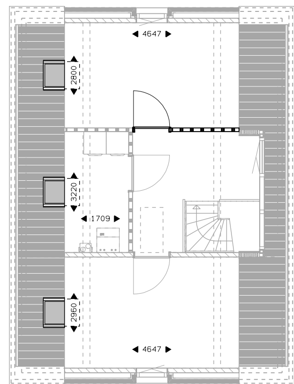
Verdieping 2 slaapkamer. dakvenster. sparing dakvenster.
