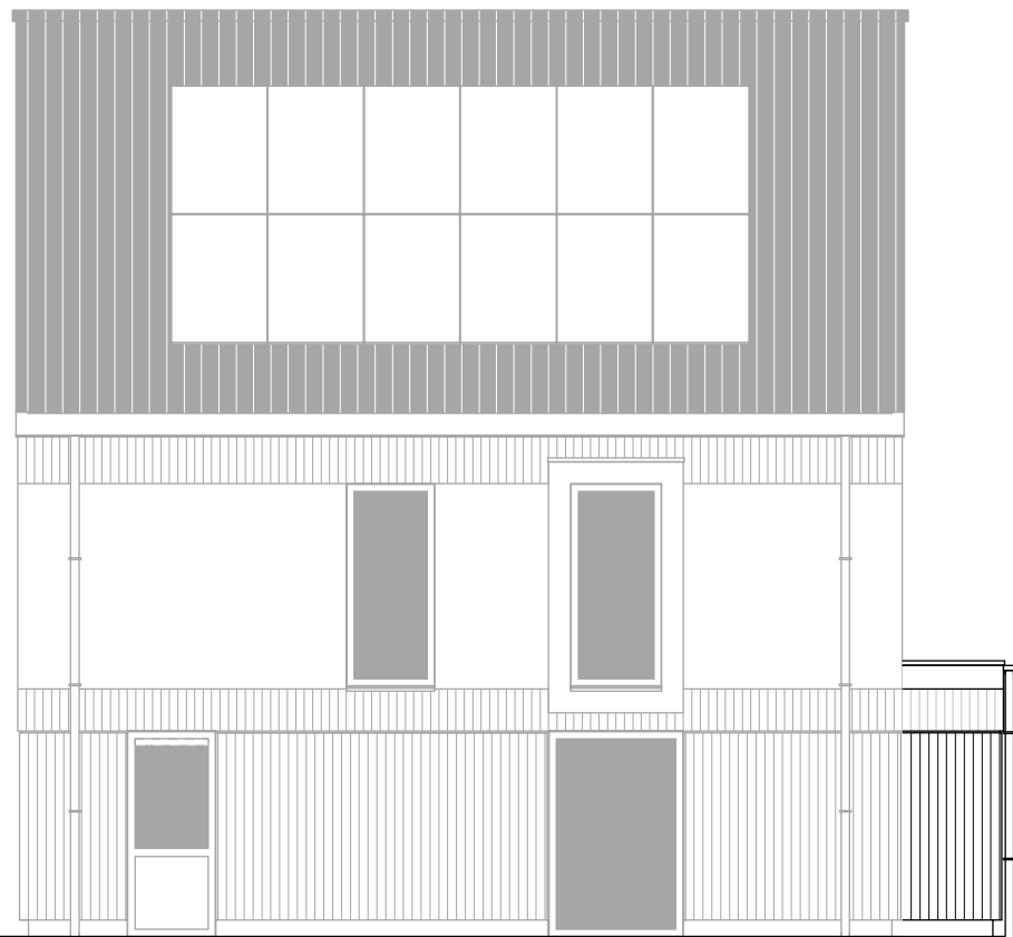
Zijgevel rechts uitbouw 1200mm.
