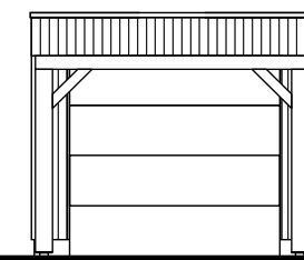
Vorgevel uitbouw 2400mm.
