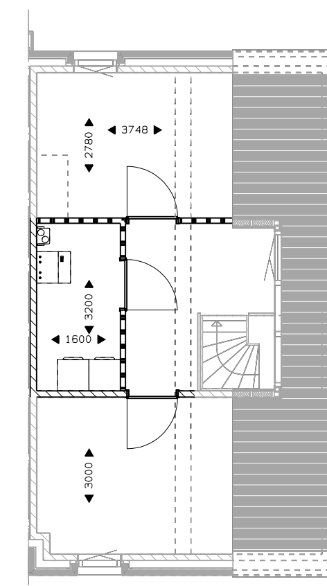
Verdieping 2 slaapkamer.
