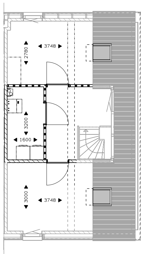
verdieping 2 slaapkamer. dakvenster. sparing dakvenster.
