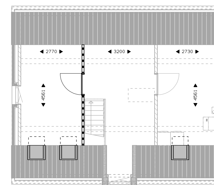
Verdieping 2 slaapkamer. dakvenster. sparing dakvenster.
