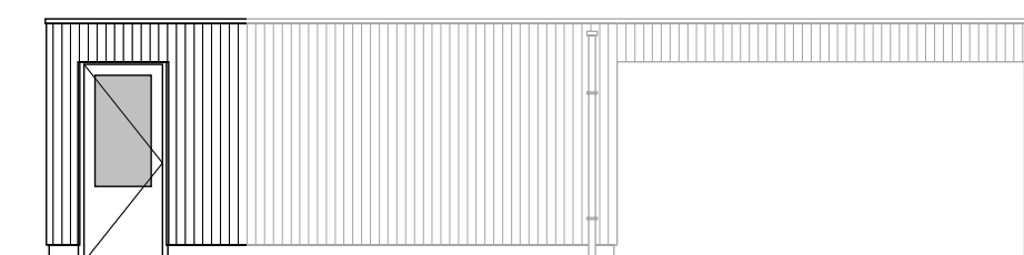
Zijgevel links uitbouw 2400mm. glasopening borstwering ca. 90 cm.
