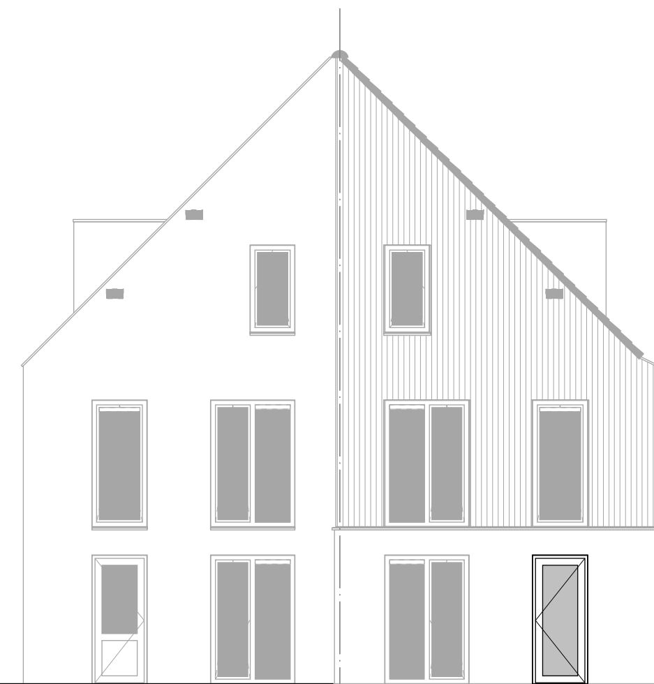
Achtergevel deur lage borstwering.
