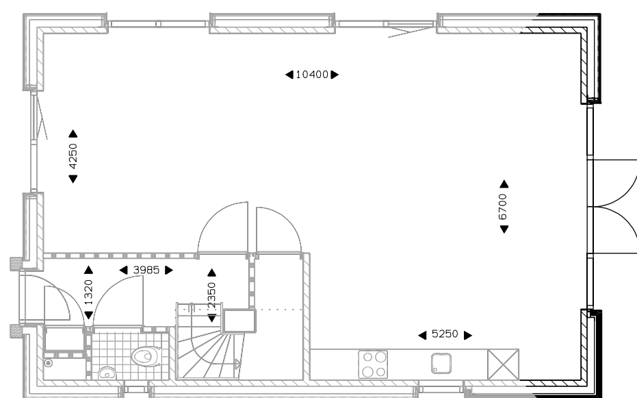
Begane grond uitbouw 1200mm *. dubbele tuindeur.
