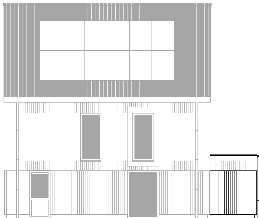
Zijgevel rechts uitbouw 2400mm.
