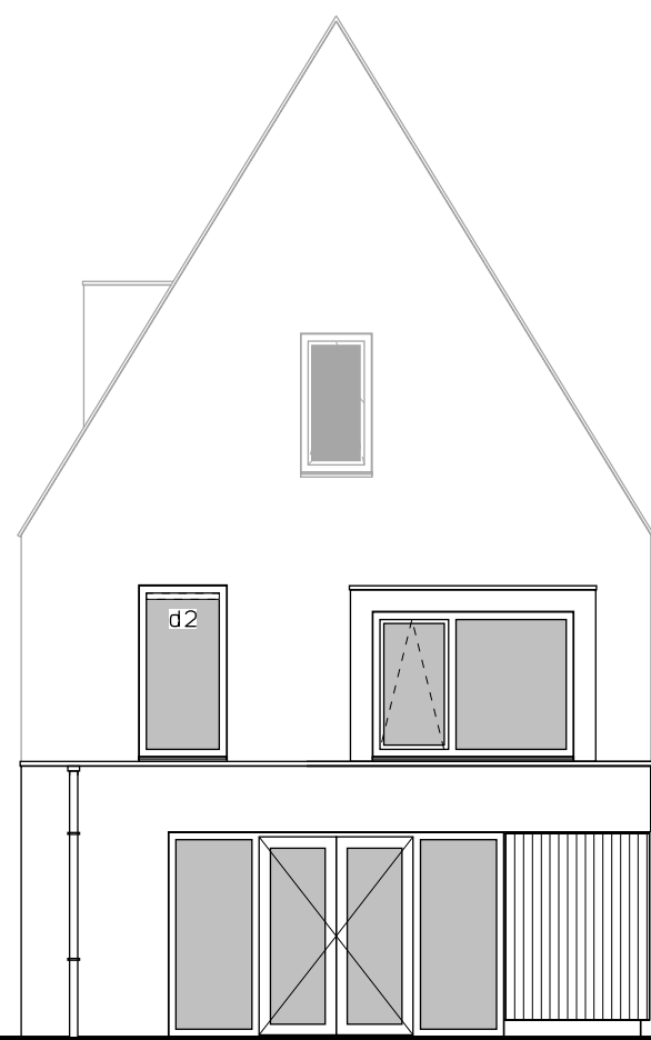
Achtergevel uitbouw 1200mm *. dubbele tuindeur.
