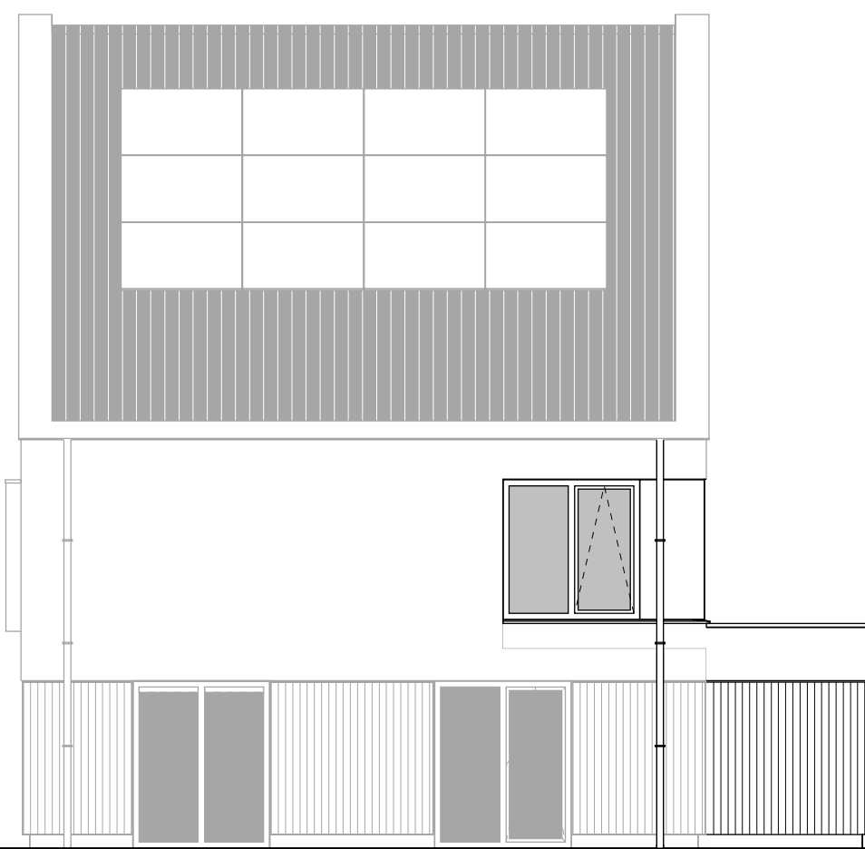
Zijgevel rechts uitbouw 2400mm.
