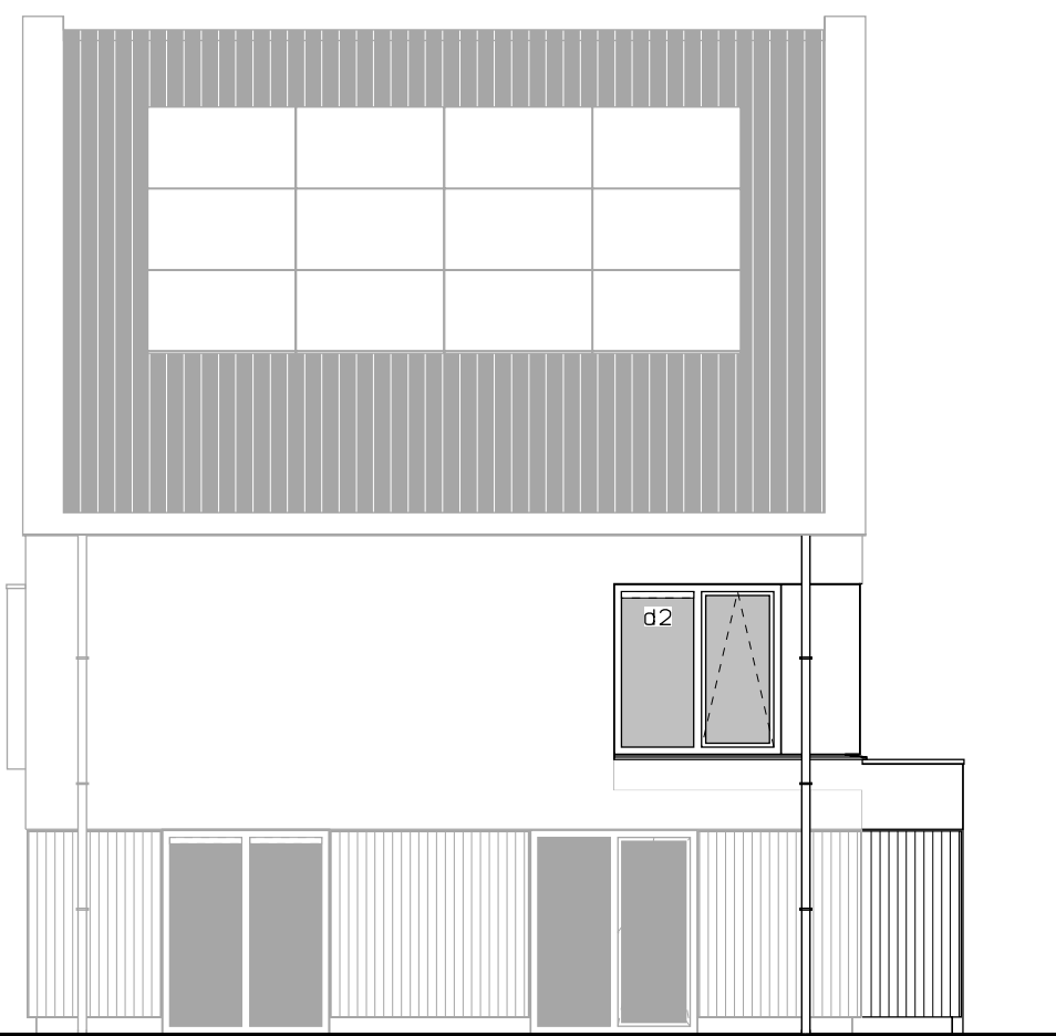
Zijgevel rechts uitbouw 1200mm.
