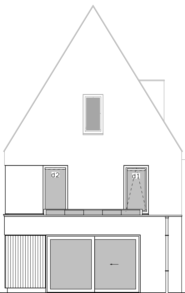
Achtergevel uitbouw 2400mm. schuifpui. lichtstraat 3 vlakken 2,40x1 m. lichtstraat 4 vlakken 3,19x1 m. lichtstraat 5 vlakken 3,89x1 m.
