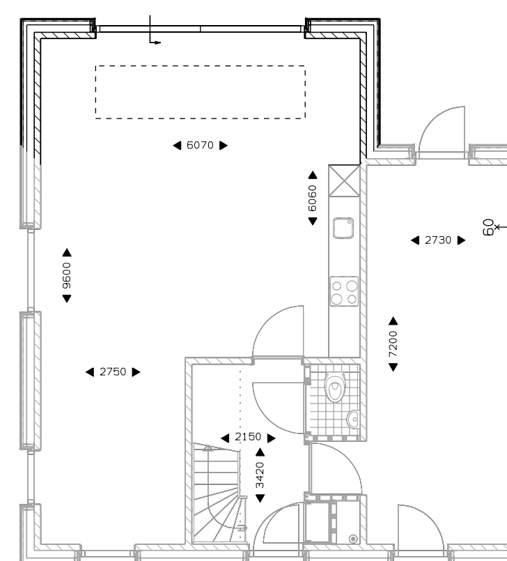
Begane grond uitbouw 2400mm. schuifpui. lichtstraat 3 vlakken 2,40x1 m. lichtstraat 4 vlakken 3,19x1 m. lichtstraat 5 vlakken 3,89x1 m.
