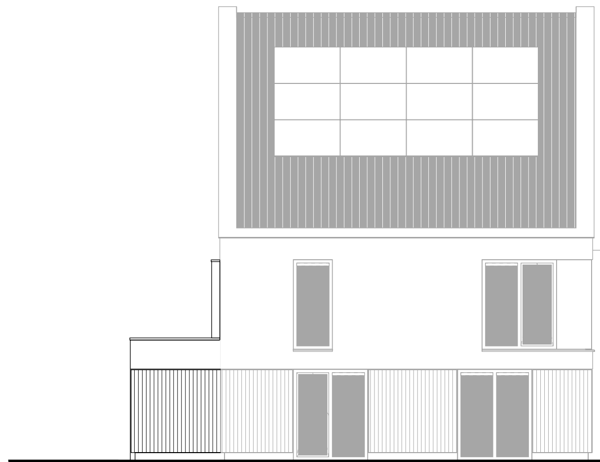
Zijgevel links uitbouw 2400mm *.
