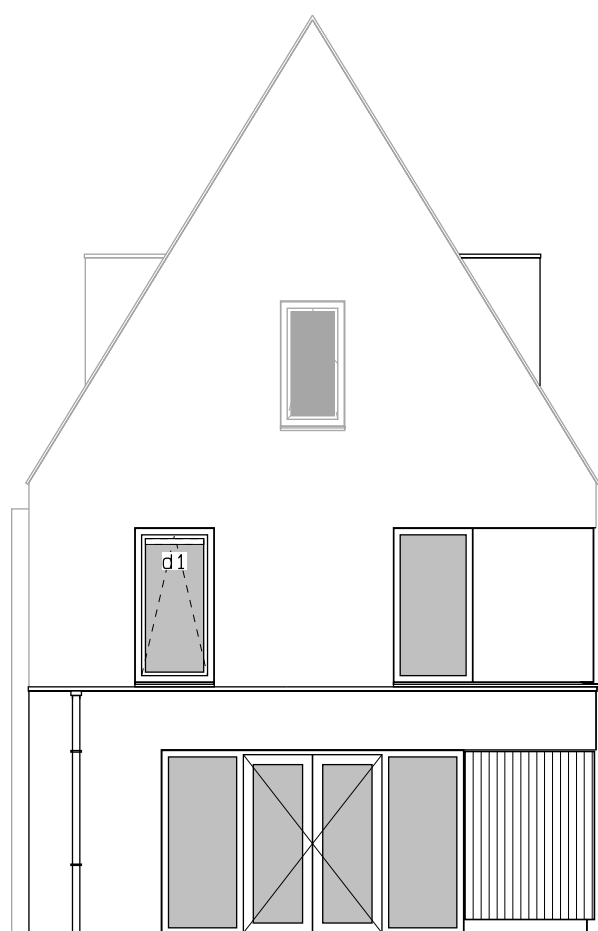
Achtergevel uitbouw 1200mm. dubbele tuindeur. dakkapel (max. 1/dakvlak). sparing dakkapel (max. 1/dakvlak).
