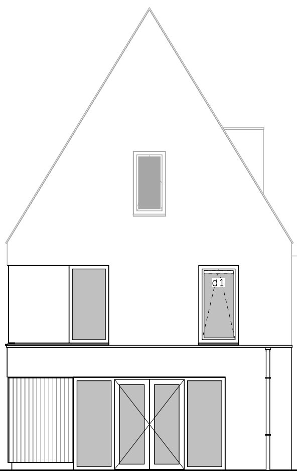
Achtergevel uitbouw 1200mm. dubbele tuindeur.
