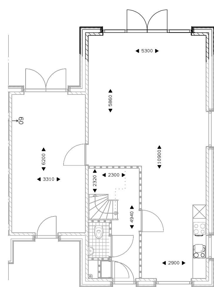
Begane grond uitbouw 1200mm. dubbele tuindeur.
