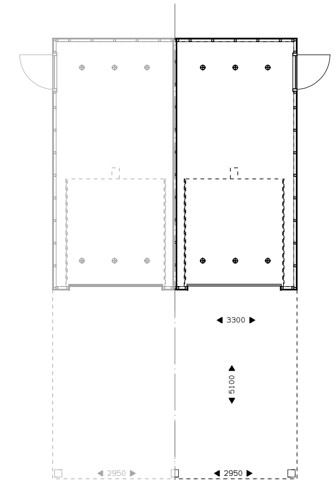
Begane grond uitbouw 2400mm. elektrisch bedienbare sectionaaldeur. natuurlijke ventilatie.
