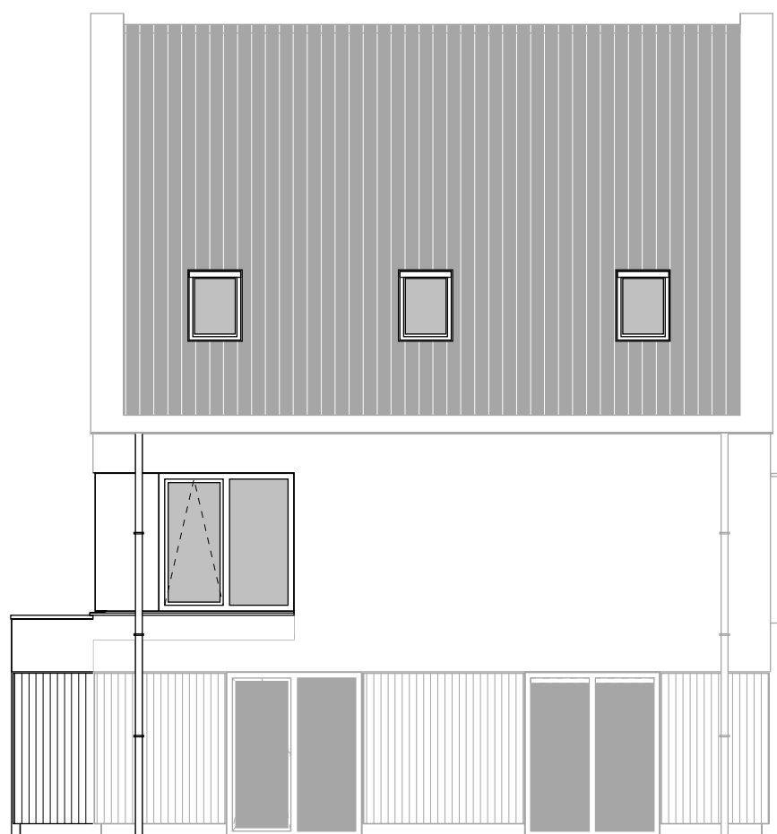
Zijgevel links uitbouw 1200mm. dakvenster. sparing dakvenster.
