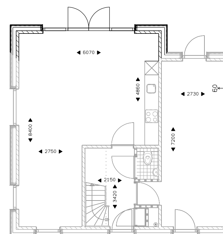
Begane grond uitbouw 1200mm.
