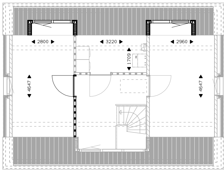
Verdieping 2 slaapkamer. dakkapel (max. 1/dakvlak). sparing dakkapel (max. 1/dakvlak).
