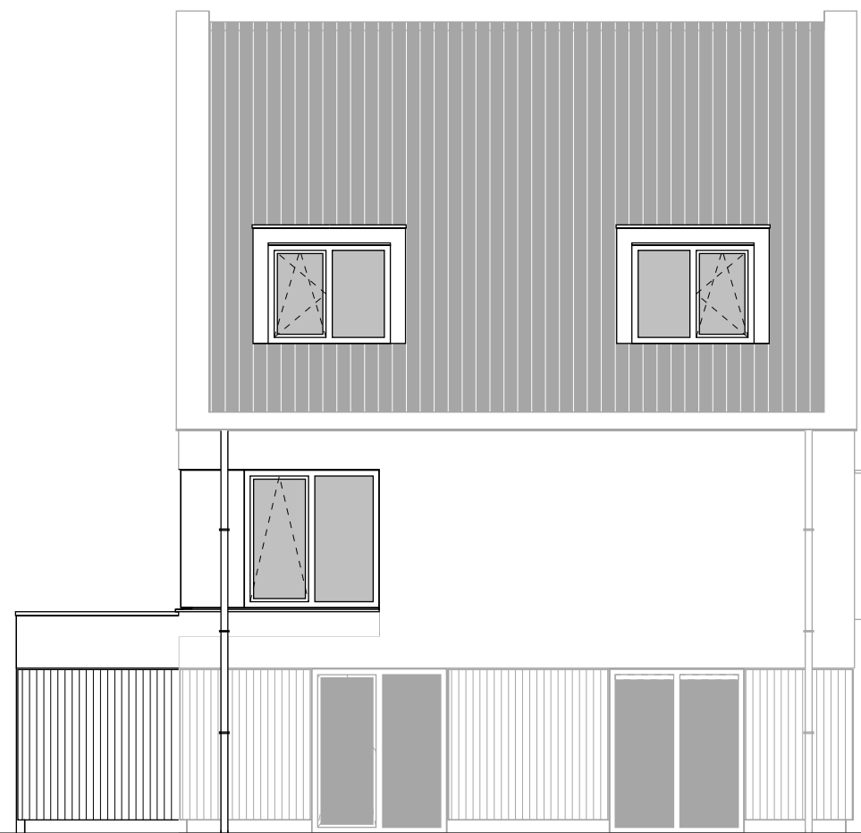
Zijgevel links uitbouw 2400mm. dakkapel (max. 1/dakvlak). sparing dakkapel (max. 1/dakvlak).
