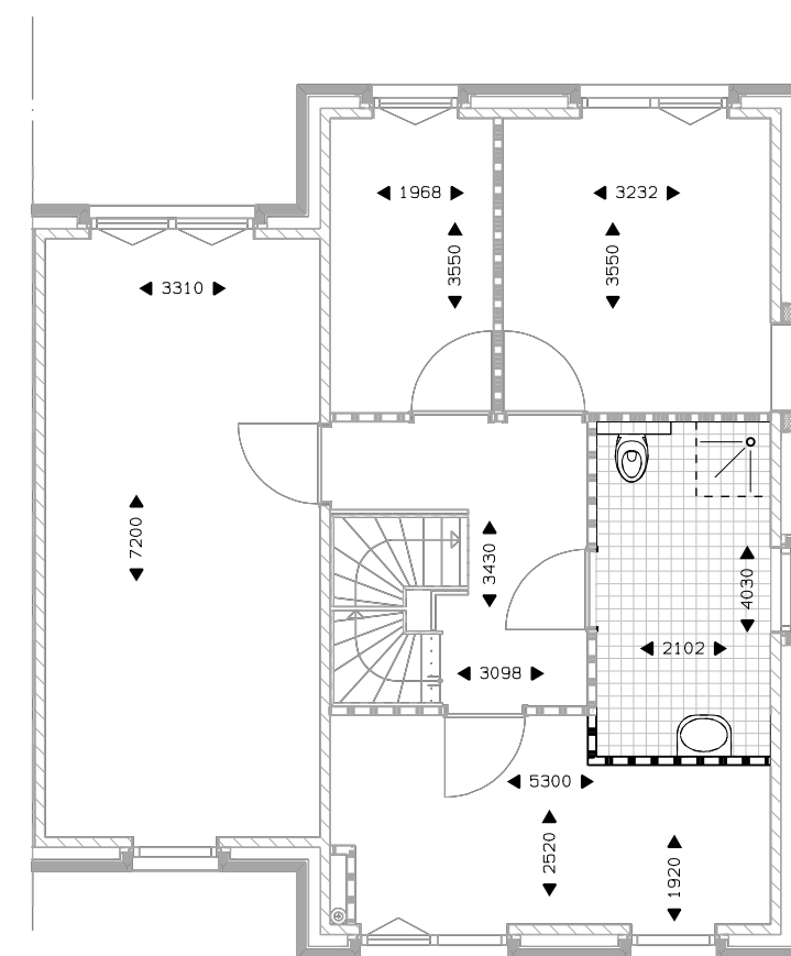
Verdieping 1 vergroten badkamer met 60 cm.
