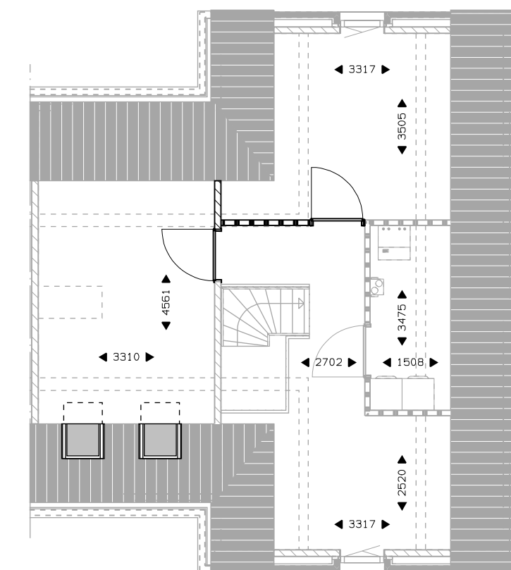
Verdieping 2 slaapkamer. dakvenster. sparing dakvenster.
