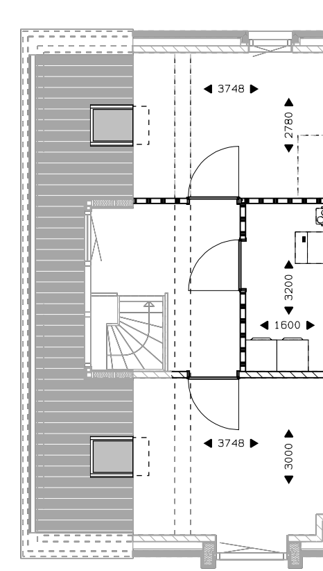
verdieping 2 slaapkamer. dakvenster. sparing dakvenster.
