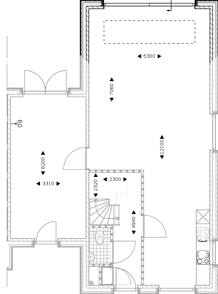
Begane grond uitbouw 2400mm. schuifpui. lichtstraat 3 vlakken 2,40x1 m. lichtstraat 4 vlakken 3,19x1 m. lichtstraat 5 vlakken 3,89x1 m.
