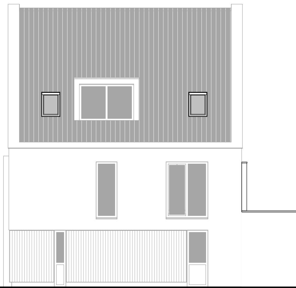
Zijgevel rechts uitbouw 2400mm *. dakvenster. sparing dakvenster.
