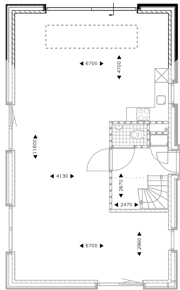
Begane grond uitbouw 2400mm. schuifpui. lichtstraat 3 vlakken 2,40x1 m. lichtstraat 4 vlakken 3,19x1 m. lichtstraat 5 vlakken 3,89x1 m.
