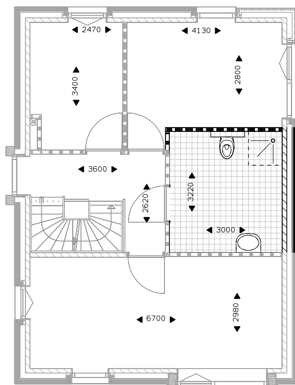
Verdieping 1 vergroten badkamer met 60 cm.
