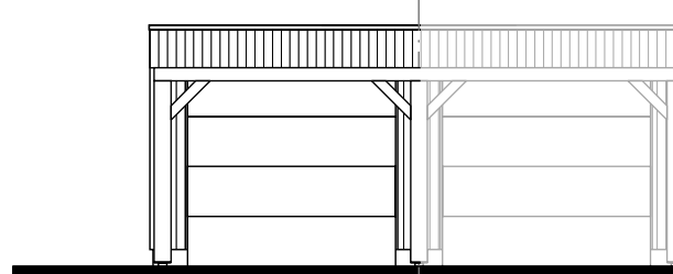
Voorgevel uitbouw 2400mm.
