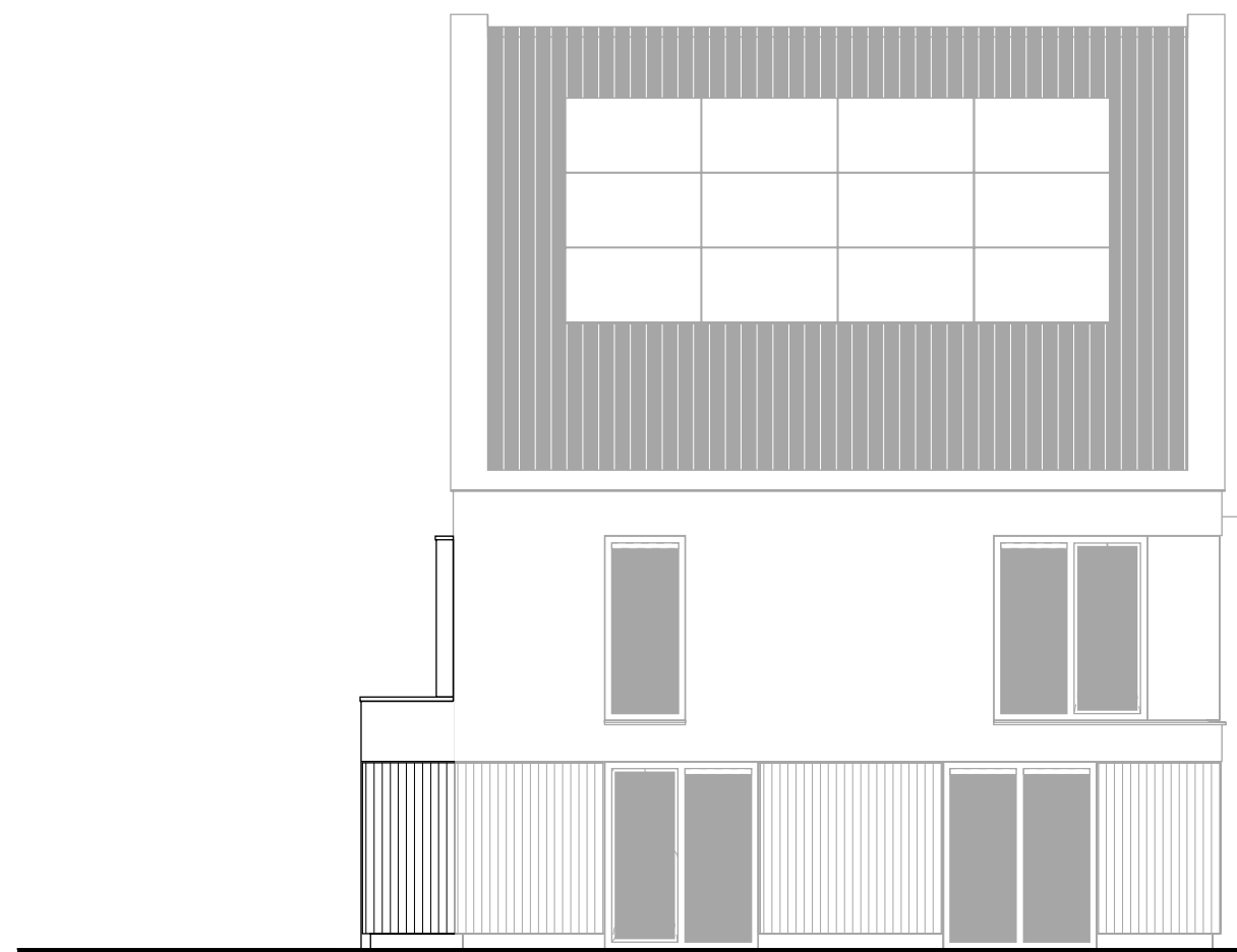
Zijgevel links uitbouw 1200mm *.
