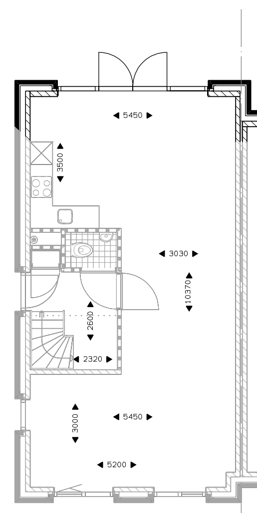
Begane grond uitbouw 1200mm. dubbele tuindeur.
