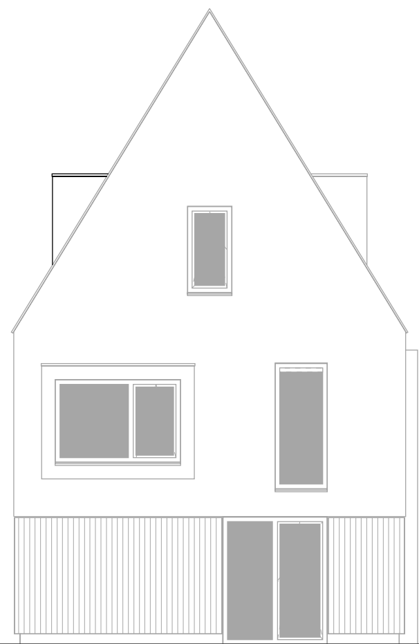
Voorgevel dakkapel (max. 1/dakvlak). sparing dakkapel (max. 1/dakvlak).
