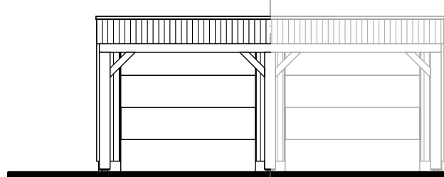
Voorgevel uitbouw 2400mm.
