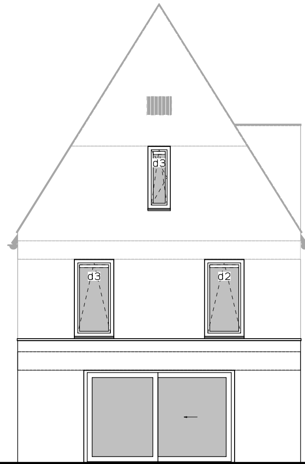
Achtergevel uitbouw 1700mm *. schuifpui.
