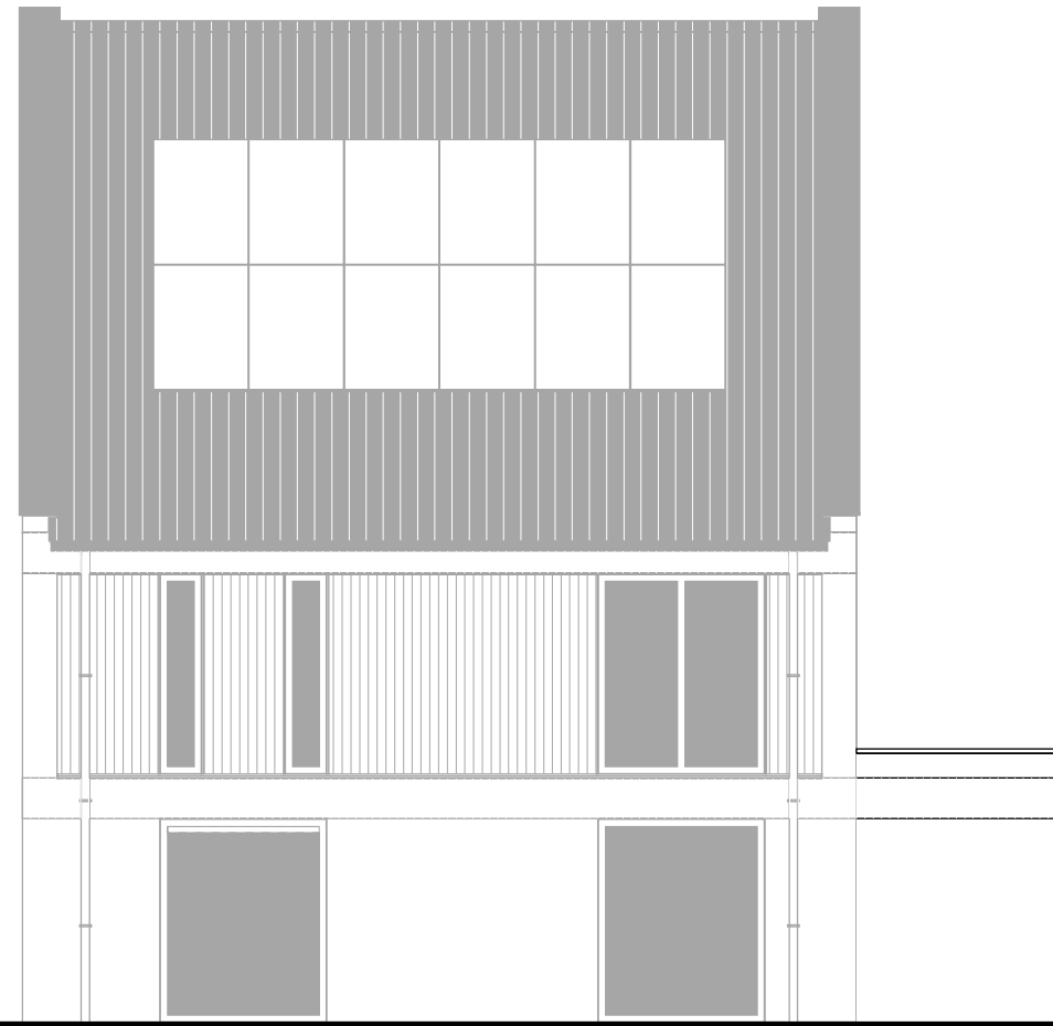
Zijgevel rechts uitbouw 1700mm *.
