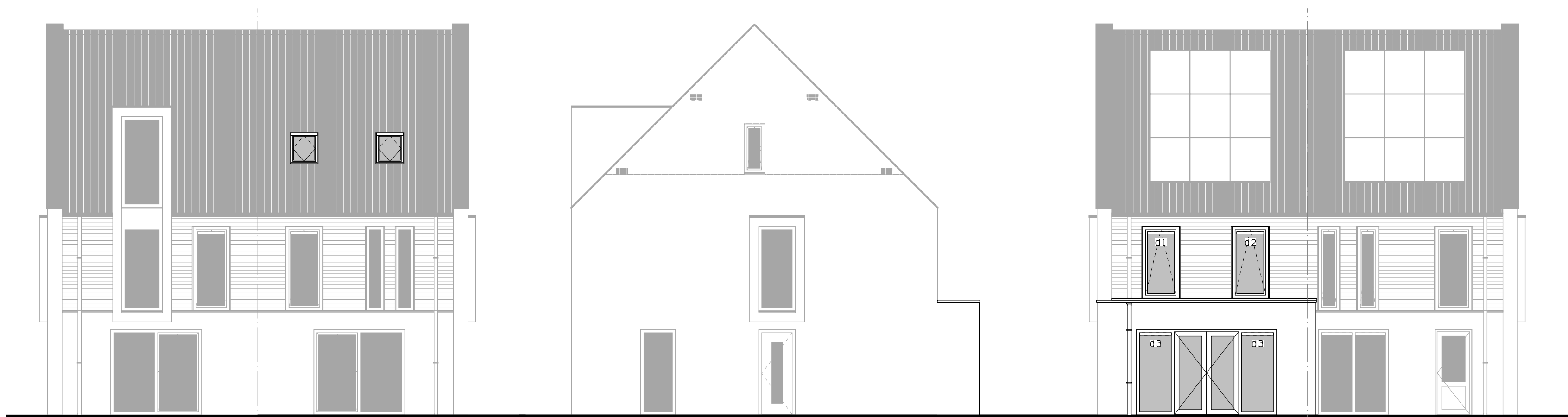
Voorgevel dakvenster. sparing dakvenster.
