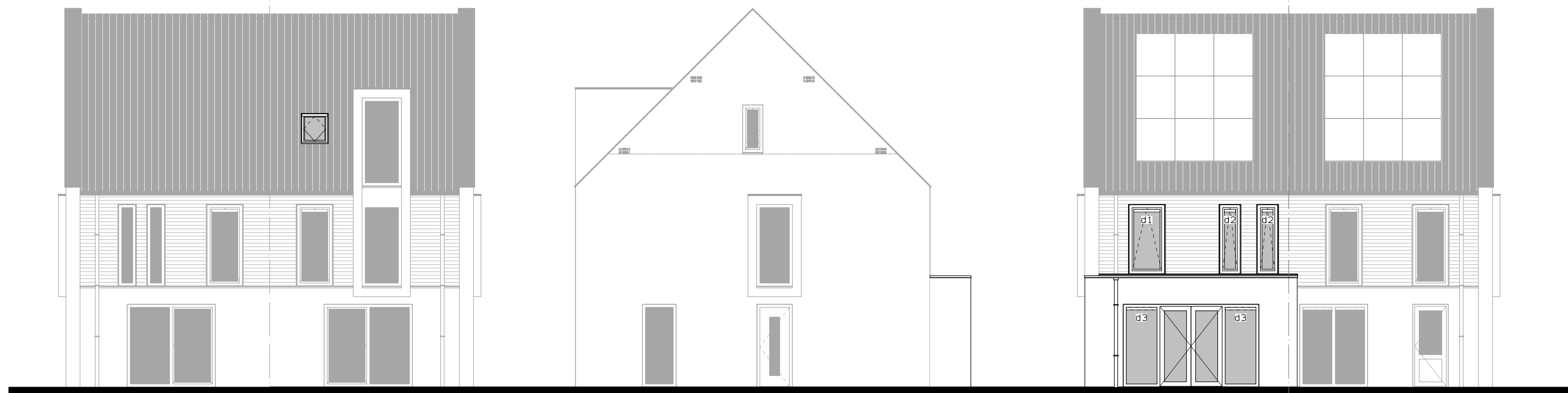
Voorgevel dakvenster. sparing dakvenster.
