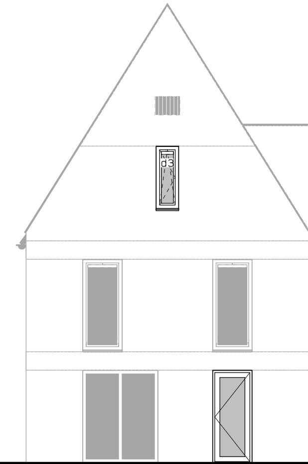
Achtergevel deur lage borstwering.
