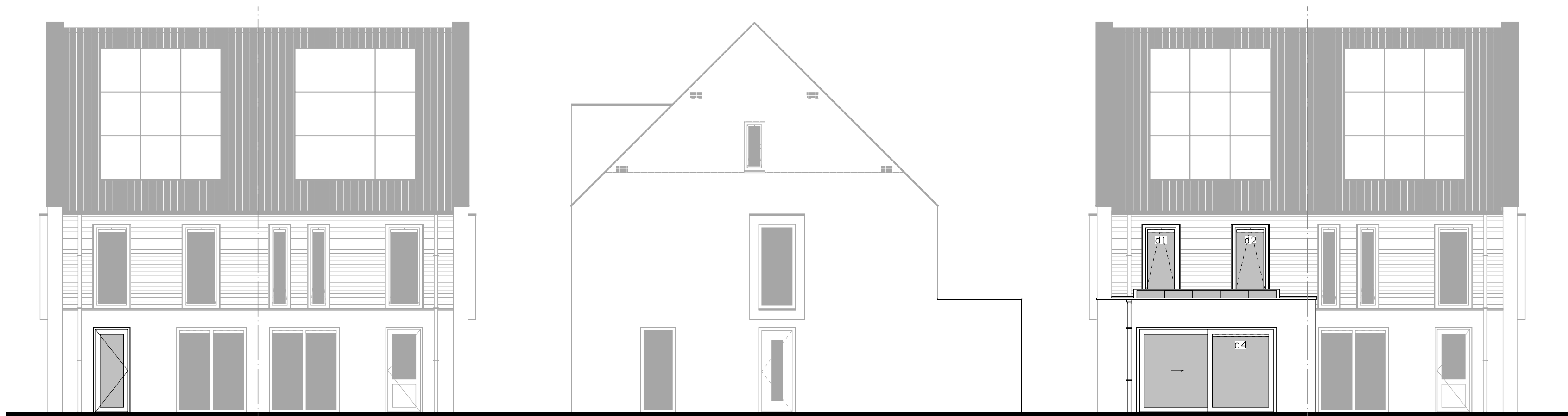
Achtergevel deur lage borstwering.
