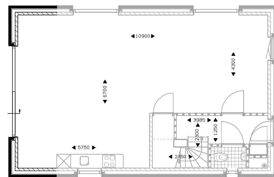
Begane grond uitbouw 1700mm *. schuifpui.
