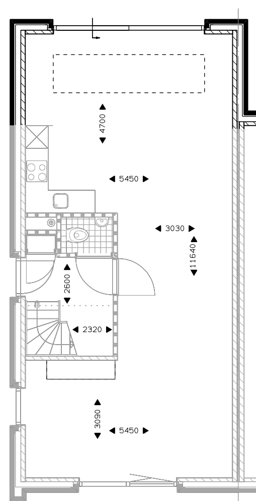
Begane grond uitbouw 2400mm. schuifpui. lichtstraat 3 vlakken 2,40x1 m. lichtstraat 4 vlakken 3,19x1 m. lichtstraat 5 vlakken 3,89x1 m.
