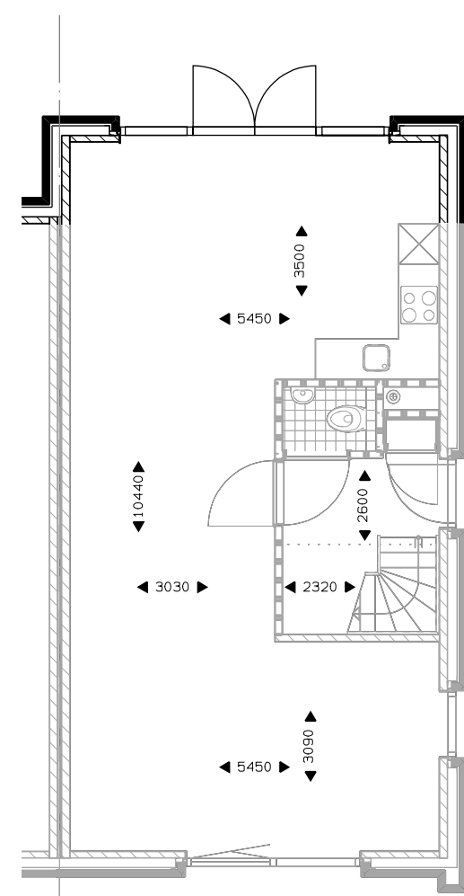
Begane grond uitbouw 1200mm. dubbele tuindeur.
