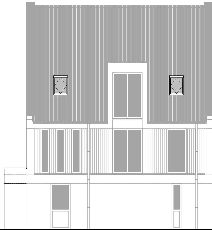
Zijgevel links uitbouw 1200mm *. dakvenster. sparing dakvenster.
