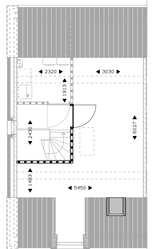
Verdieping 2 slaapkamer. dakvenster. sparing dakvenster.
