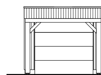
Voorgevel uitbouw 2400mm.
