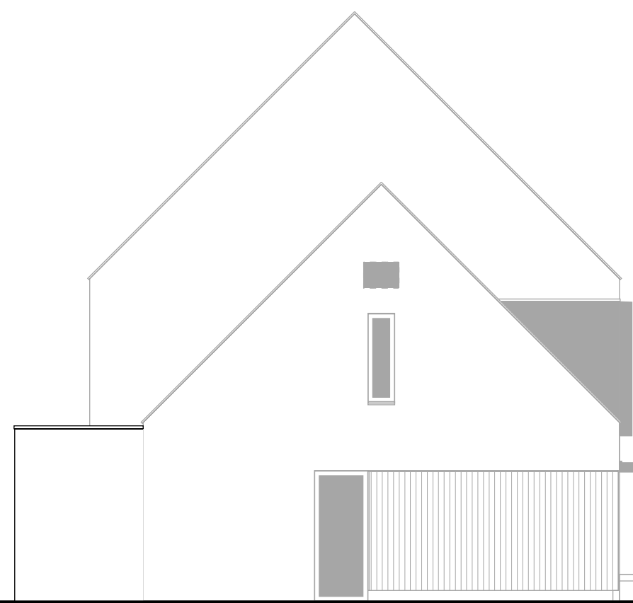
Zijgevel links uitbouw 2400mm.
