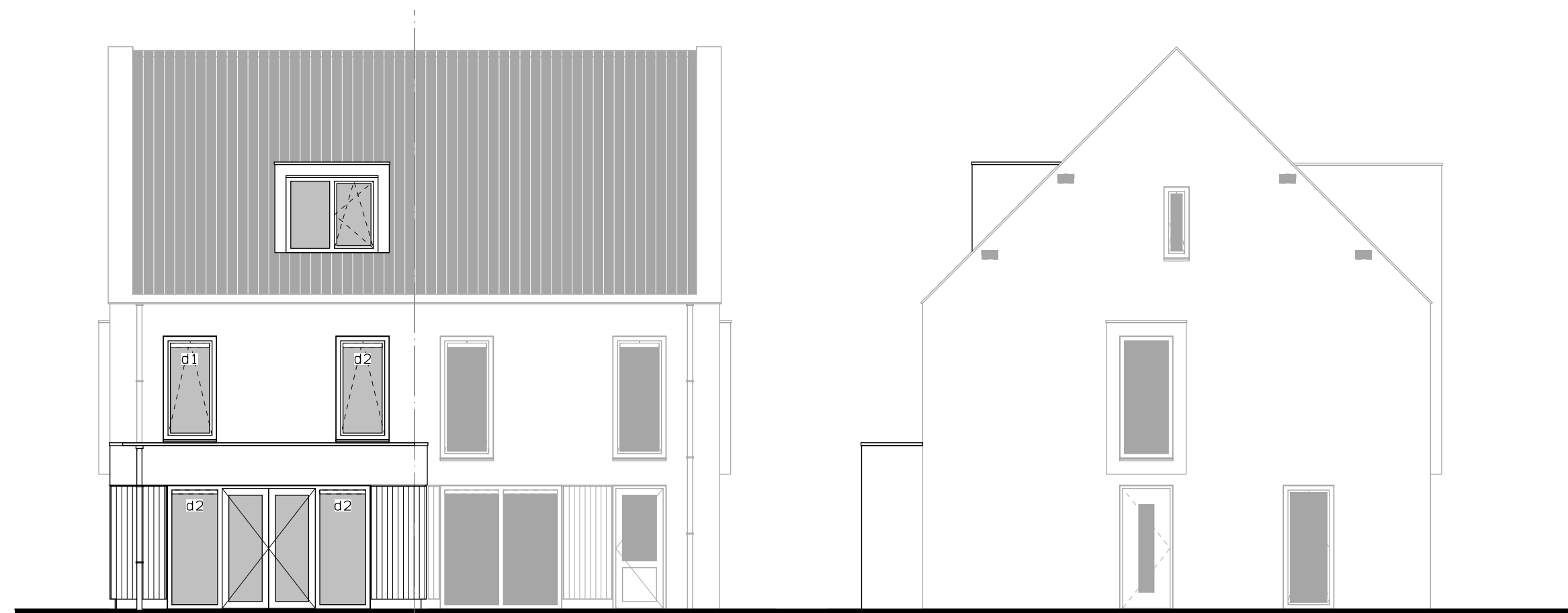
Achtergevel uitbouw 1200mm. dubbele tuindeur. dakkapel (max. 1/dakvlak). sparing dakkapel (max. 1/dakvlak).
