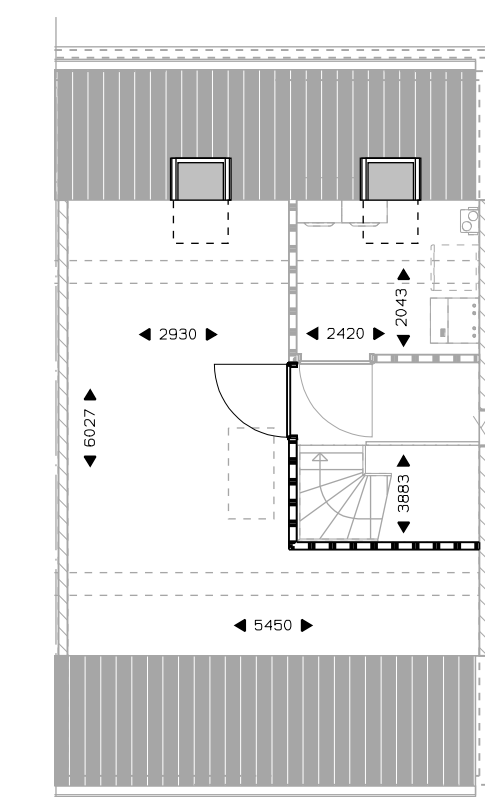
Verdieping 2 slaapkamer. dakvenster. sparing dakvenster.
