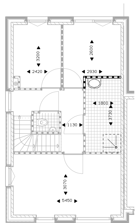
Verdieping 1 vergroten badkamer met 60 cm.
