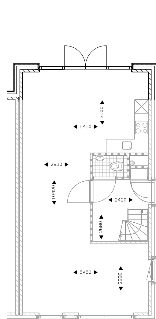
Begane grond uitbouw 1200mm. dubbele tuindeur.
