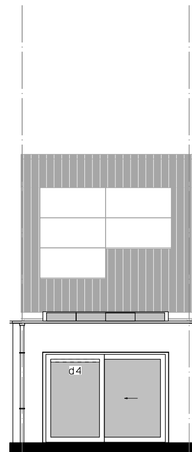
Achtergevel uitbouw 2400mm. schuifpui. lichtstraat 3 vlakken 2,40x1 m. lichtstraat 4 vlakken 3,19x1 m.
