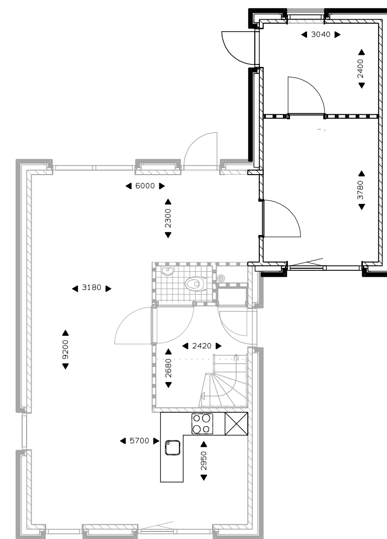
Begane grond keuken voorzijde. berging indelen in speelkamer/bijkeuken (seperate berging min. 5m² verplicht).
