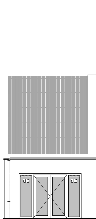
Achtergevel uitbouw 1200mm. dubbele tuindeur.
