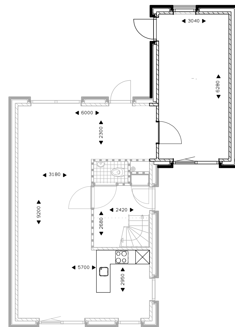
Begane grond keuken voorzijde. berging wordt speelkamer (seperate berging min. 5m² verplicht).
