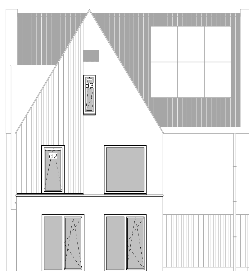
Zijgevel rechts uitbouw 1200mm *.
