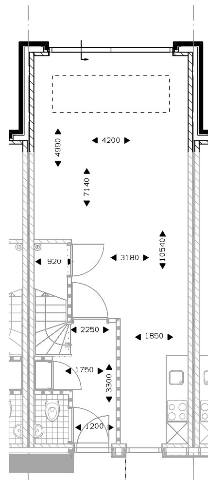
Begane grond uitbouw 2400mm. schuifpui. lichtstraat 3 vlakken 2,40x1 m. lichtstraat 4 vlakken 3,19x1 m.
