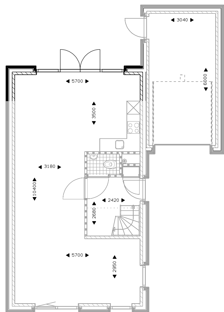
Begane grond uitbouw 1200mm. dubbele tuindeur. berging isoleren.
