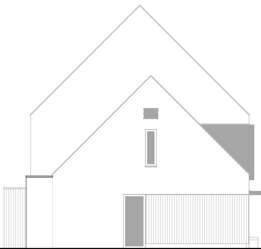
Zijgevel links uitbouw 1200mm.
