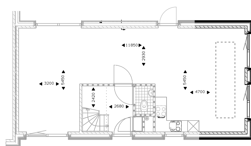
Begane grond uitbouw 2400mm *. schuifpui. lichtstraat 3 vlakken 2,40x1 m. lichtstraat 4 vlakken 3,19x1 m. lichtstraat 5 vlakken 3,89x1 m.
