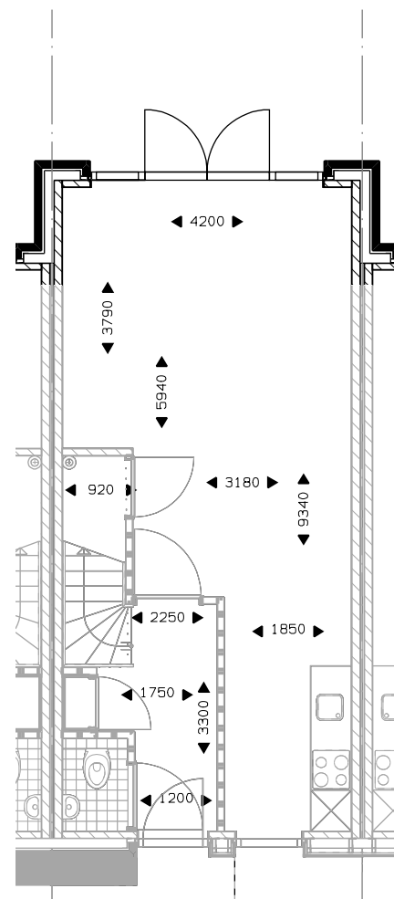
Begane grond uitbouw 1200mm. dubbele tuindeur.
