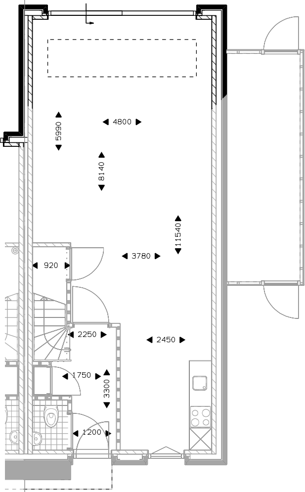
Begane grond uitbouw 2400mm. schuifpui. lichtstraat 3 vlakken 2,40x1 m. lichtstraat 4 vlakken 3,19x1 m. lichtstraat 5 vlakken 3,89x1 m.
