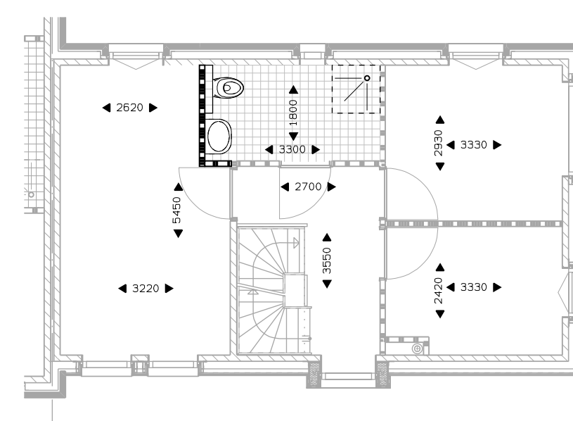
Verdieping 1 vergroten badkamer met 60 cm.
