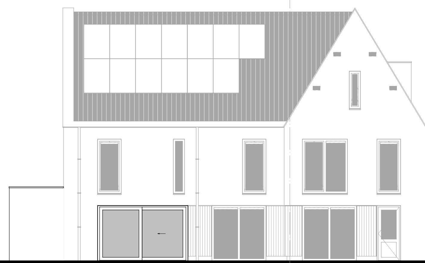
Achtergevel uitbouw 2400mm *. schuifpui.
