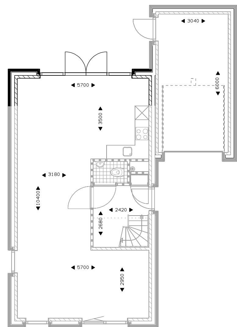
Begane grond uitbouw 1200mm. dubbele tuindeur. berging isoleren.
