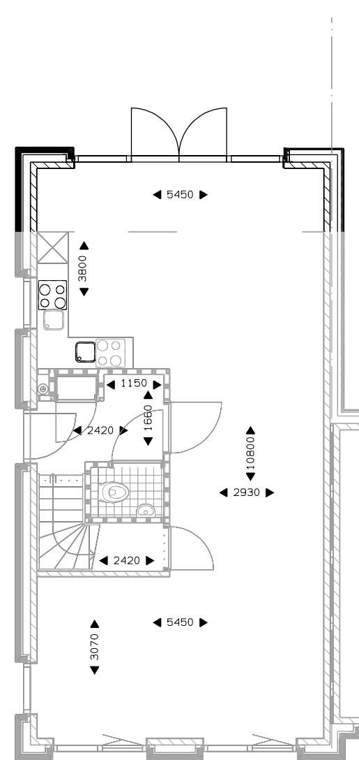
Begane grond uitbouw 1200mm. dubbele tuindeur.
