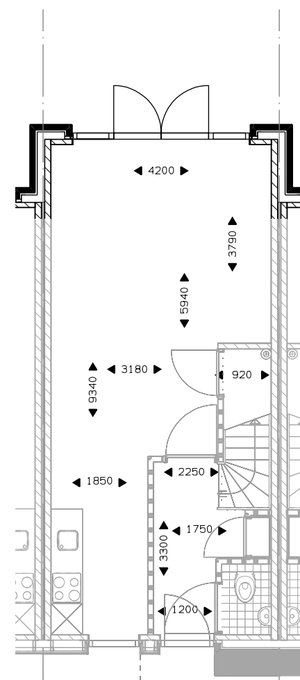
Begane grond uitbouw 1200mm. dubbele tuindeur.
