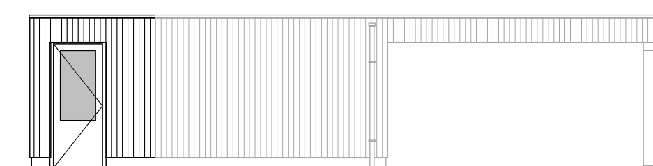
Zijgevel links uitbouw 2400mm. glasopening borstwering ca. 90 cm.
