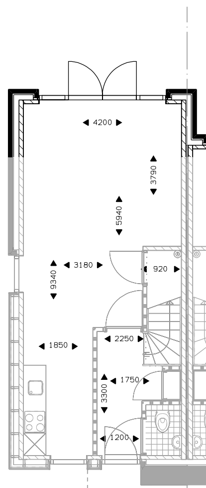
Begane grond uitbouw 1200mm. dubbele tuindeur.
