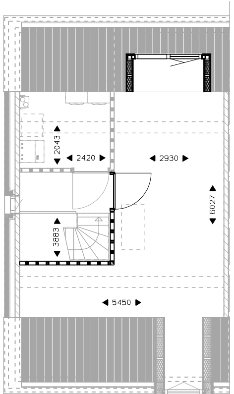
Verdieping 2 slaapkamer. dakkapel (max. 1/dakvlak). sparing dakkapel (max. 1/dakvlak).
