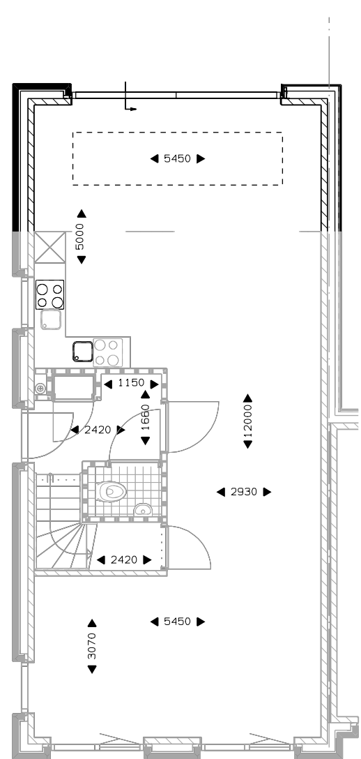
Begane grond uitbouw 2400mm. schuifpui. lichtstraat 3 vlakken 2,40x1 m. lichtstraat 4 vlakken 3,19x1 m. lichtstraat 5 vlakken 3,89x1 m.
