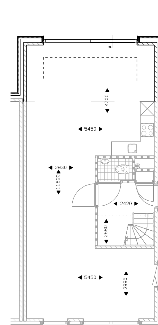
Begane grond uitbouw 2400mm. schuifpui. lichtstraat 3 vlakken 2,40x1 m. lichtstraat 4 vlakken 3,19x1 m. lichtstraat 5 vlakken 3,89x1 m.
