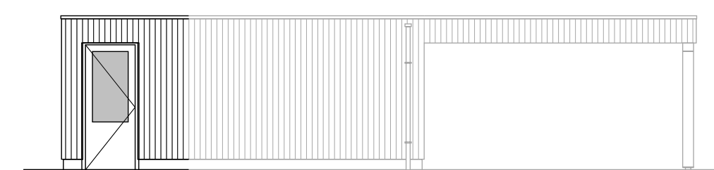
Zijgevel links uitbouw 2400mm. glasopening borstwering ca. 90 cm.
