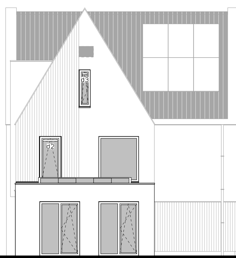
Zijgevel rechts uitbouw 2400mm *. lichtstraat 3 vlakken 2,40x1 m. lichtstraat 4 vlakken 3,19x1 m. lichtstraat 5 vlakken 3,89x1 m.
