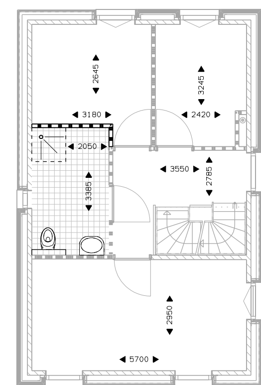
Verdieping 1 vergroten badkamer met 60 cm.
