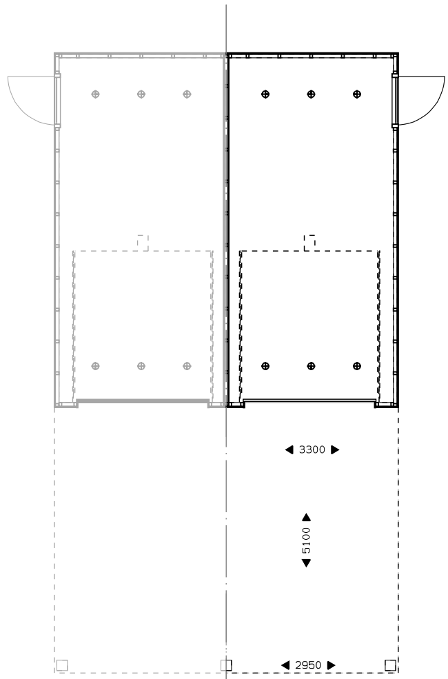
Begane grond uitbouw 2400mm. elektrisch bedienbare sectionaaldeur. natuurlijke ventilatie.
