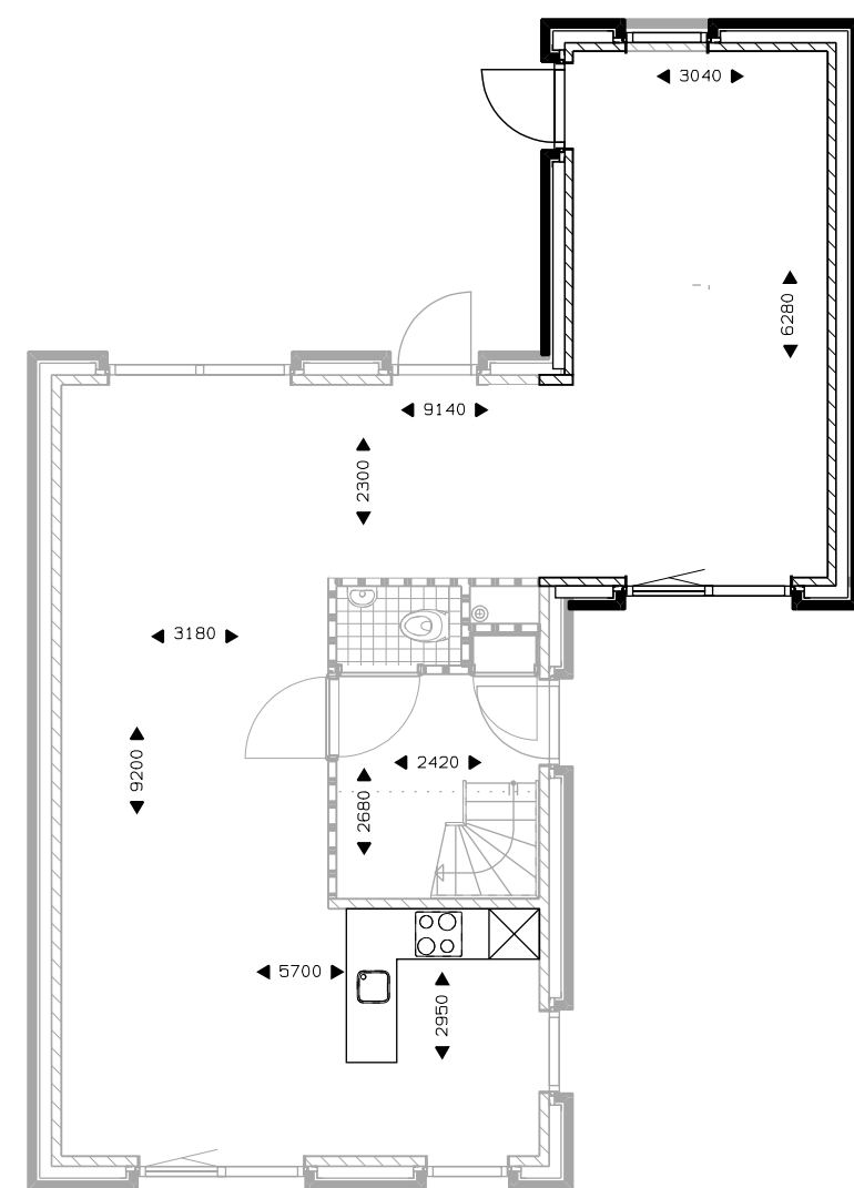
Begane grond keuken voorzijde. berging betrekken bij woning (seperate berging min. 5m² verplicht).
