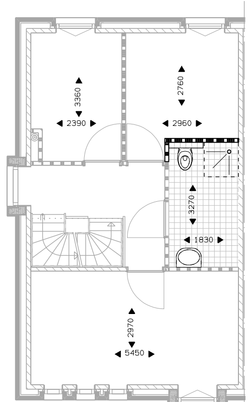
Verdieping 1 vergroten badkamer met 60 cm.
