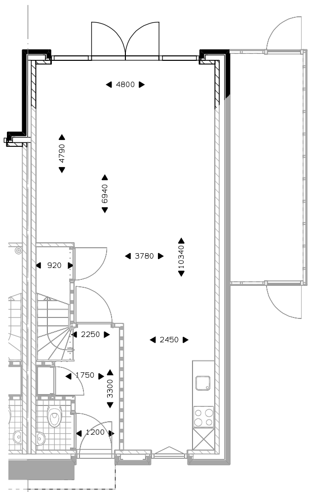
Begane grond uitbouw 1200mm. dubbele tuindeur.
