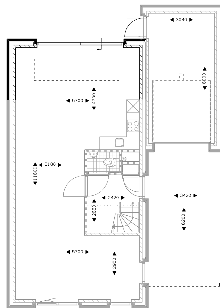
Begane grond uitbouw 2400mm. schuifpui. lichtstraat 3 vlakken 2,40x1 m. lichtstraat 4 vlakken 3,19x1 m. lichtstraat 5 vlakken 3,89x1 m. carport.
