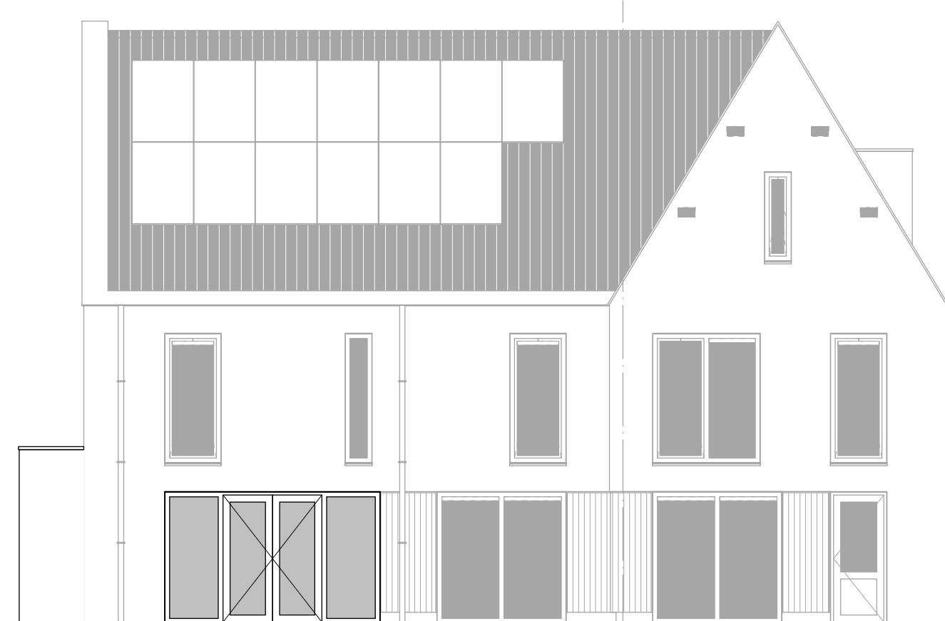
Achtergevel uitbouw 1200mm *. dubbele tuindeur.
