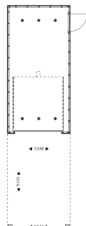
Begane grond uitbouw 2400mm. elektrisch bedienbare sectionaaldeur. natuurlijke ventilatie.
