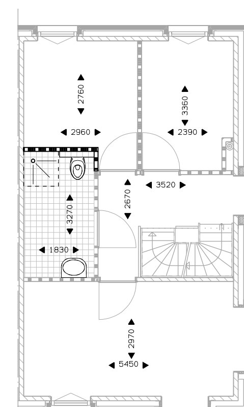
Verdieping 1 vergroten badkamer met 60 cm.
