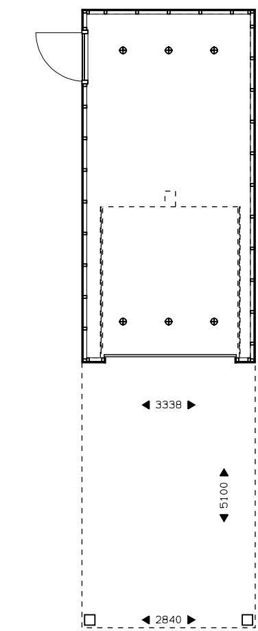
Begane grond uitbouw 2400mm. elektrisch bedienbare sectionaaldeur. natuurlijke ventilatie.
