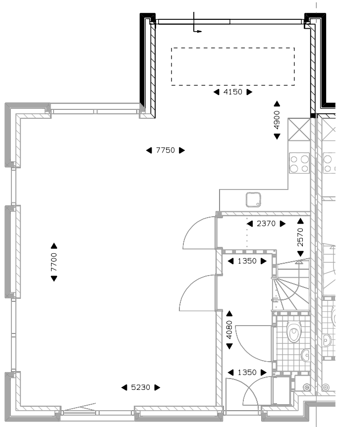
Begane grond uitbouw 2400mm. schuifpui. lichtstraat 3 vlakken 2,40x1 m. lichtstraat 4 vlakken 3,19x1 m.
