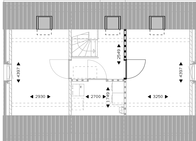
Verdieping 2 slaapkamer. dakvenster. sparing dakvenster.
