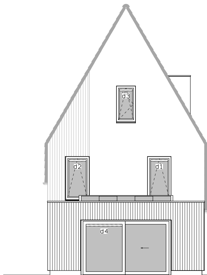
Zijgevel links uitbouw 2400mm. schuifpui. lichtstraat 3 vlakken 2,40x1 m. lichtstraat 4 vlakken 3,19x1 m. lichtstraat 5 vlakken 3,89x1 m. dakkapel (max. 1/dakvlak). sparing dakkapel (max. 1/dakvlak).
