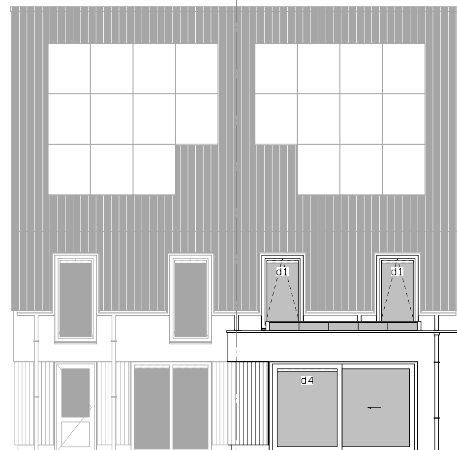
Achtergevel uitbouw 2400mm. schuifpui. lichtstraat 3 vlakken 2,40x1 m. lichtstraat 4 vlakken 3,19x1 m. lichtstraat 5 vlakken 3,89x1 m.
