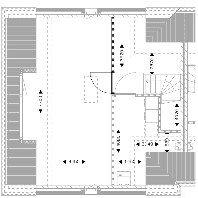
Verdieping 2 slaapkamer.
