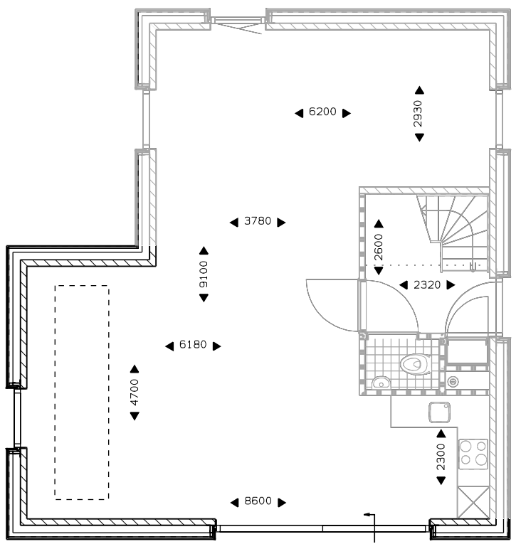
Begane grond uitbouw 2400mm. schuifpui. lichtstraat 3 vlakken 2,40x1 m. lichtstraat 4 vlakken 3,19x1 m. lichtstraat 5 vlakken 3,89x1 m.
