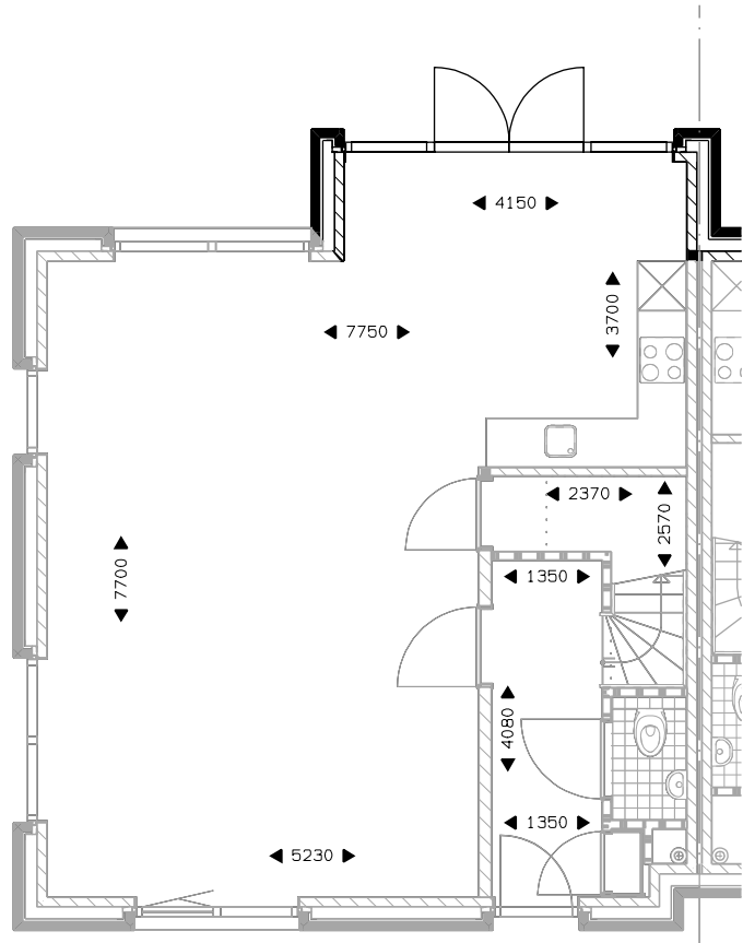
Begane grond uitbouw 1200mm. dubbele tuindeur.
