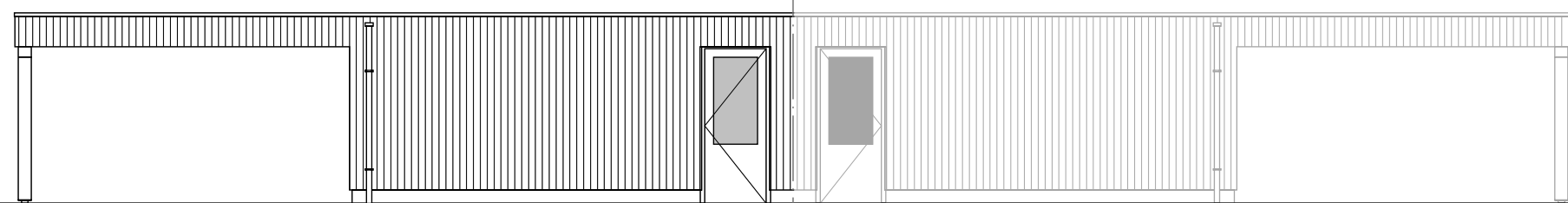
Zijgevel rechts uitbouw 2400mm. glasopening borstwering ca. 90 cm.
