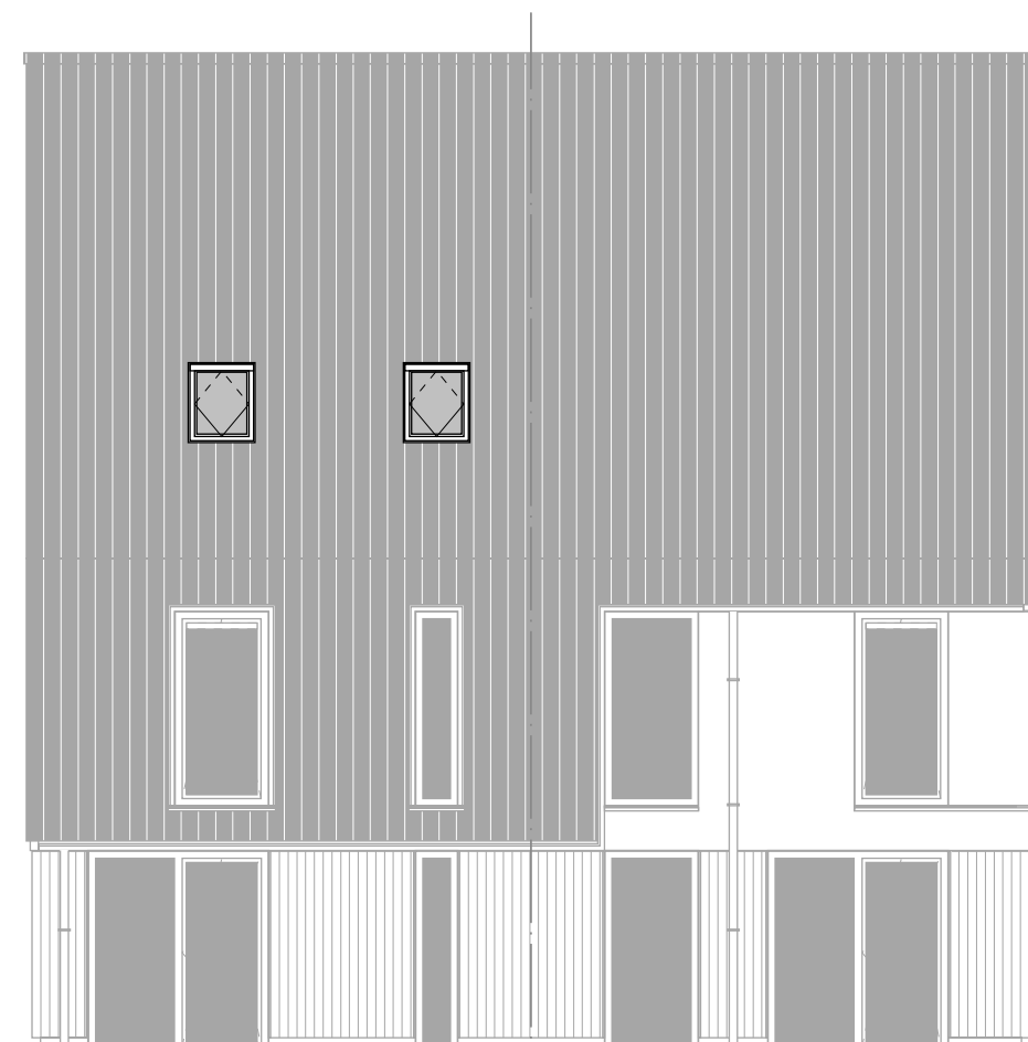
Voorgevel dakvenster. sparing dakvenster.
