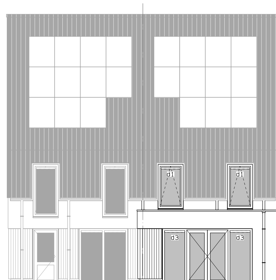
Achtergevel uitbouw 1200mm. dubbele tuindeur.
