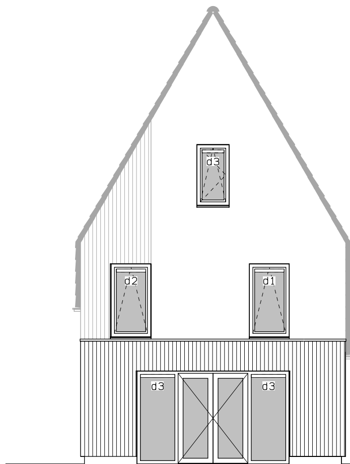
Zijgevel links uitbouw 1200mm. dubbele tuindeur.
