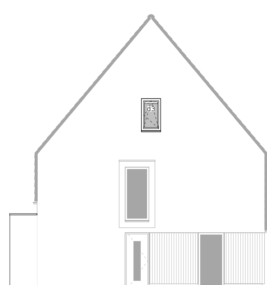
Zijgevel links uitbouw 1200mm.
