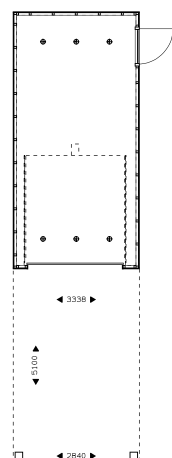
Begane grond uitbouw 2400mm. elektrisch bedienbar sectionaaldeur. natuurlijke ventilatie.
