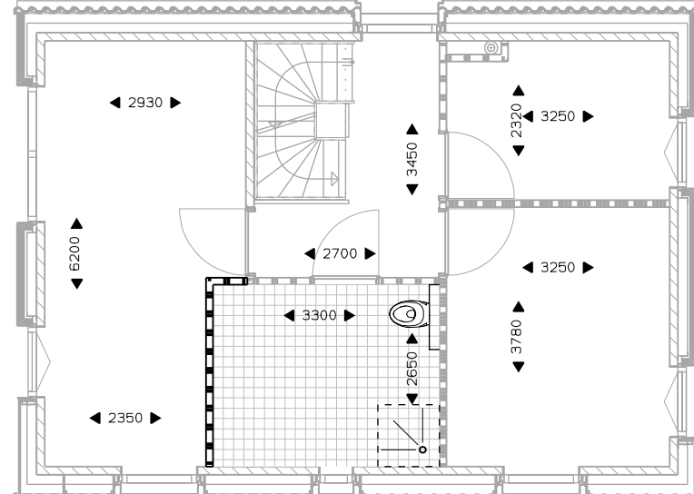
Verdieping 1 vergroten badkamer met 60 cm.
