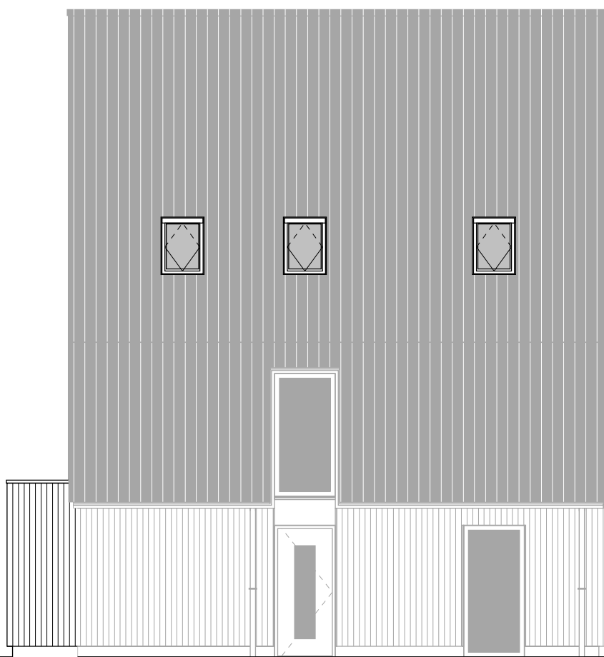
Voorgevel uitbouw 1200mm. dakvenster. sparing dakvenster.
