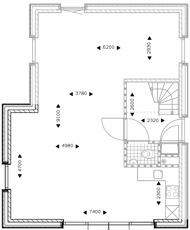
Begane grond uitbouw 1200mm. dubbele tuindeur.
