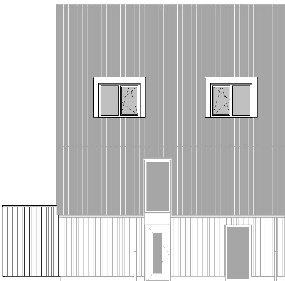
Voorgevel uitbouw 2400mm. dakkapel (max. 1/dakvlak). sparing dakkapel (max. 1/dakvlak).
