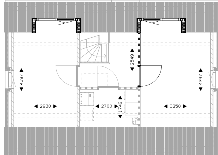
Verdieping 2 slaapkamer. dakkapel (max. 1/dakvlak). sparing dakkapel (max. 1/dakvlak).
