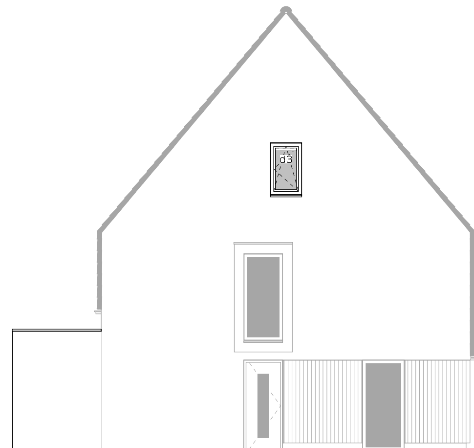
Zijgevel links uitbouw 2400mm.
